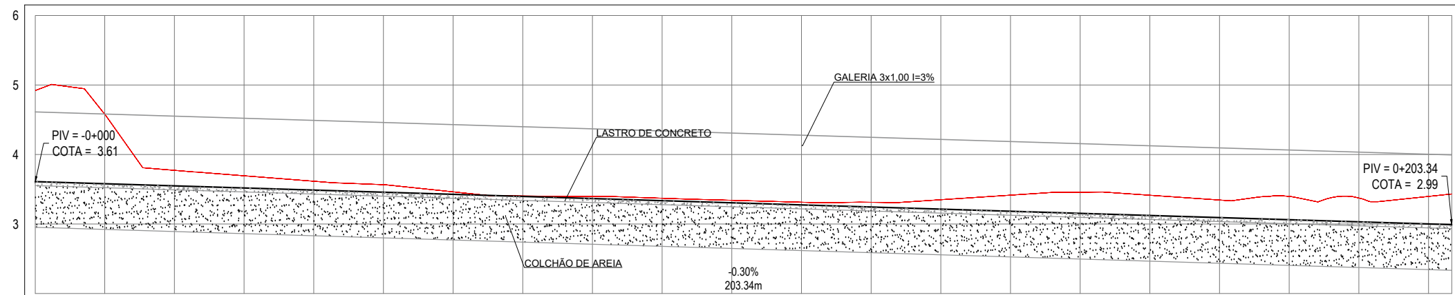
PERFIL: CANAL
