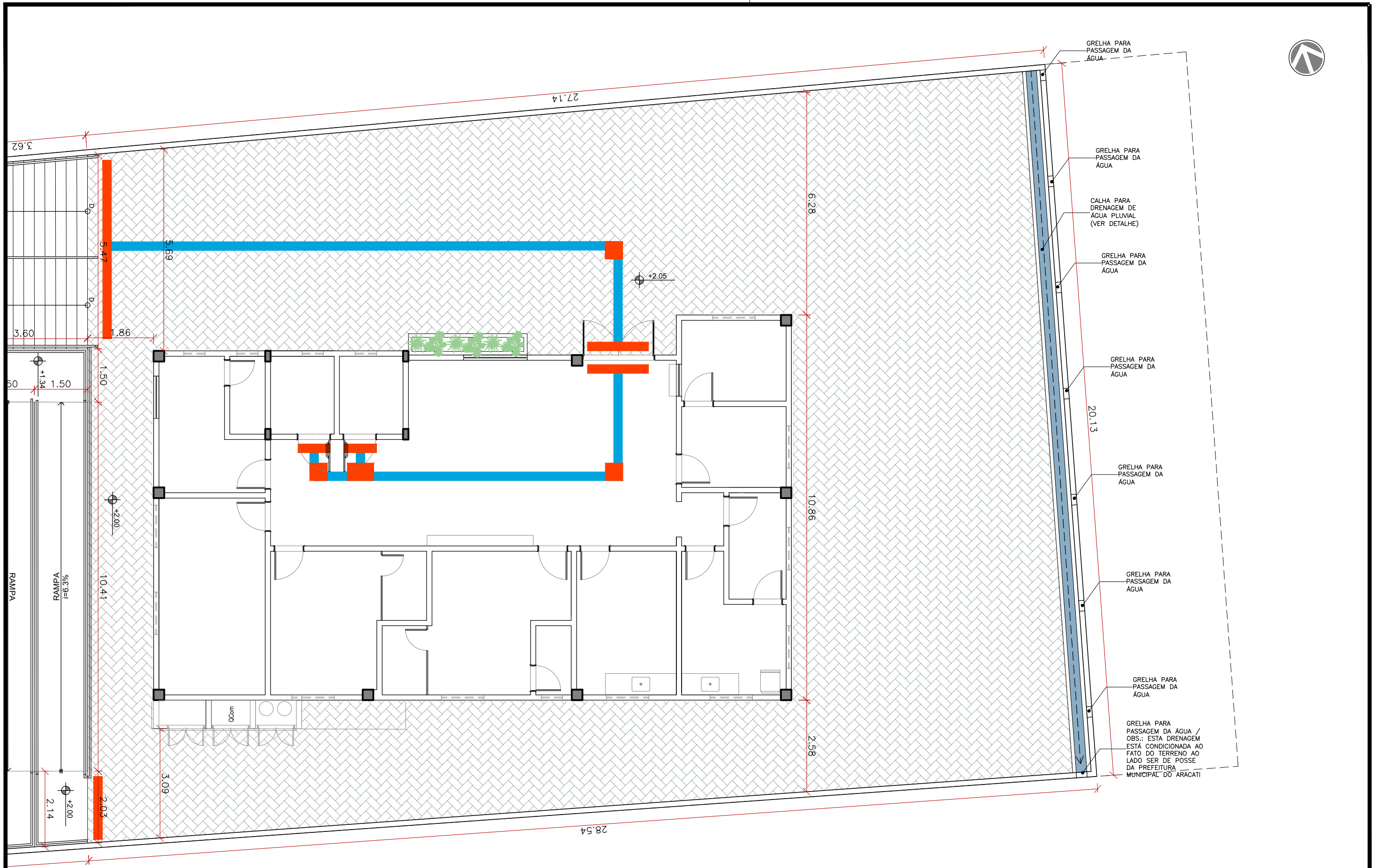
01 PLANTA - ACESSO E DRENAGEM ESCALA 1/100
