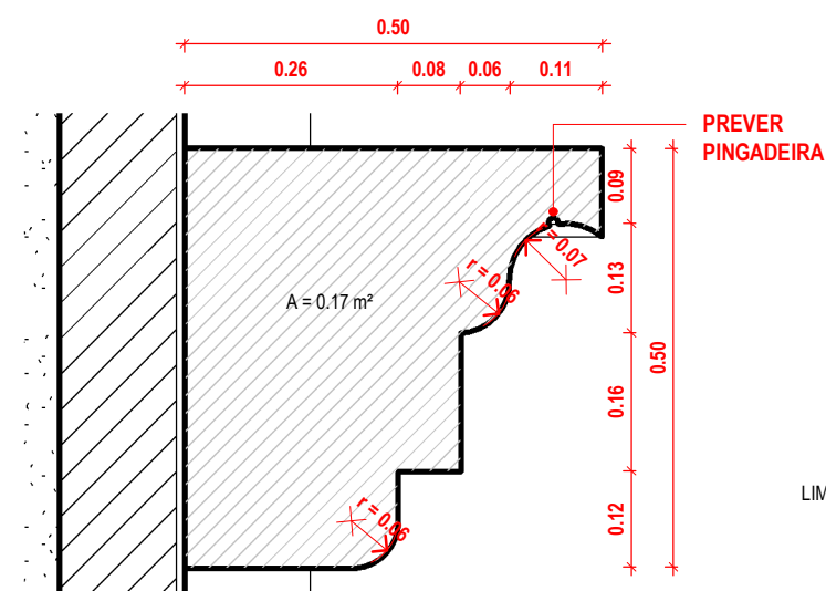
2 | DETALHE SANCA 1:10
