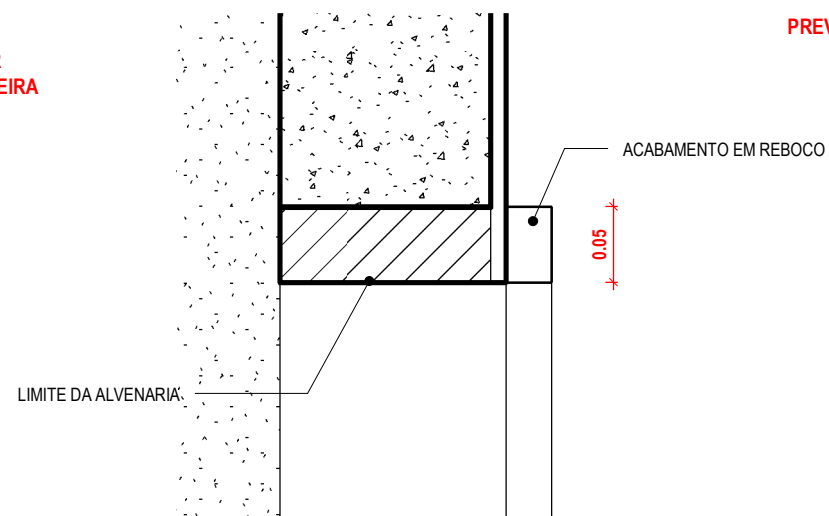
3 | DETALHE MOLDURA EM EPS 1:5
