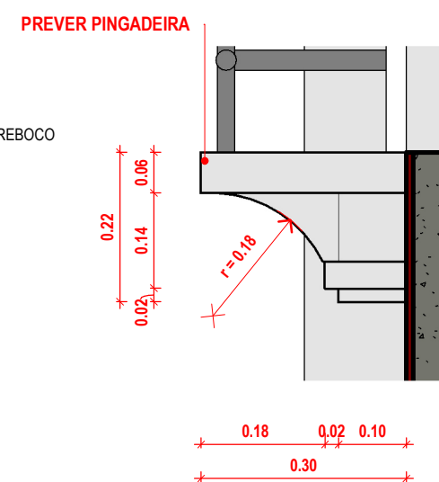
4 | DETALHE SACADA 1:10
