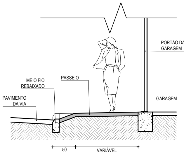
02 CORTE A-A ESCALA: SEM ESCALA
