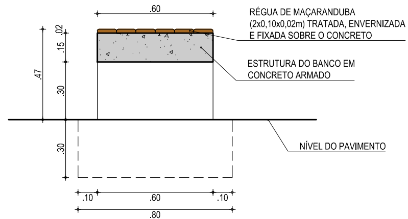
BANCO - CORTE A-A
