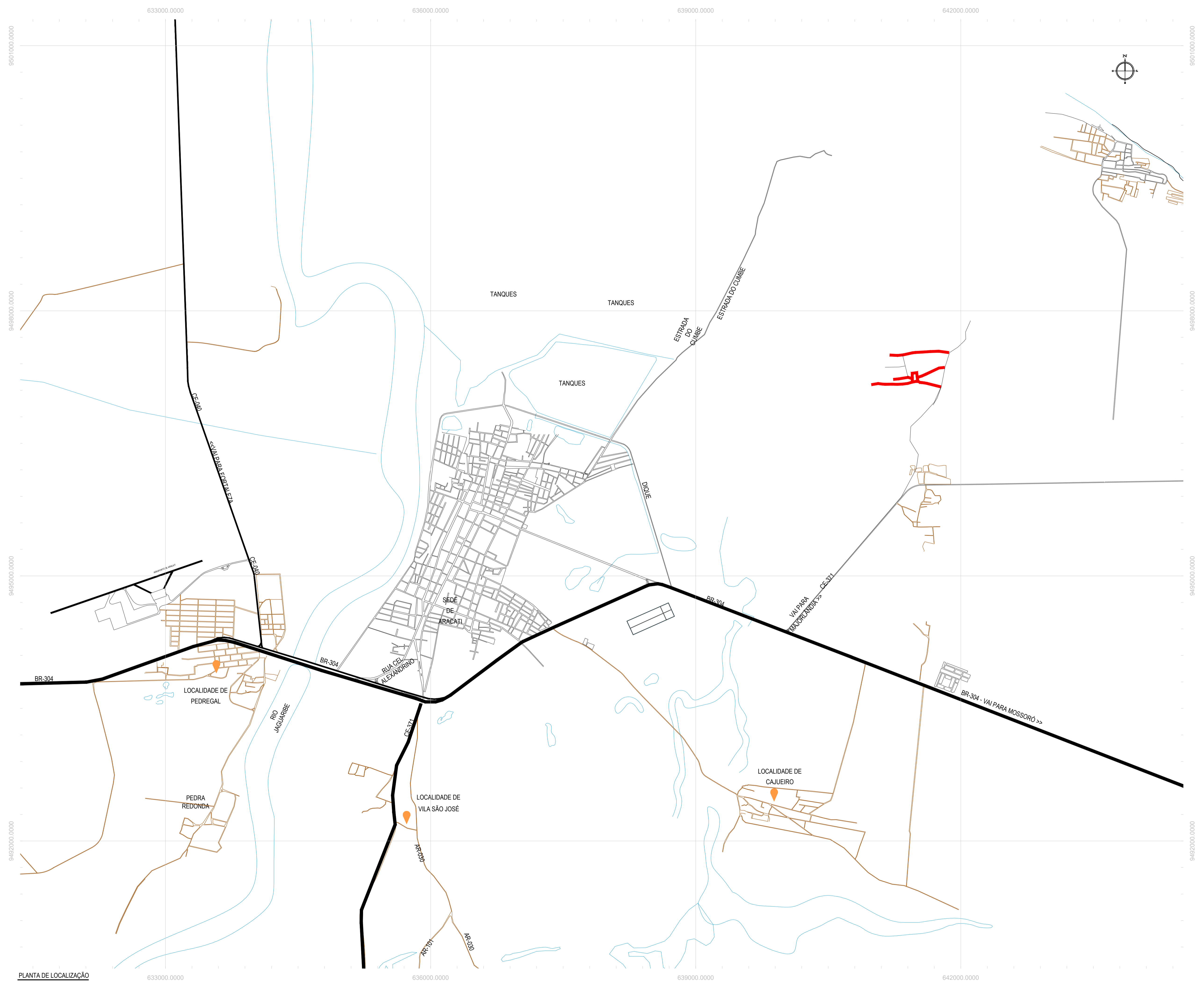
PLANTA DE LOCALIZAÇÃO ESCALA: 1:20.000
