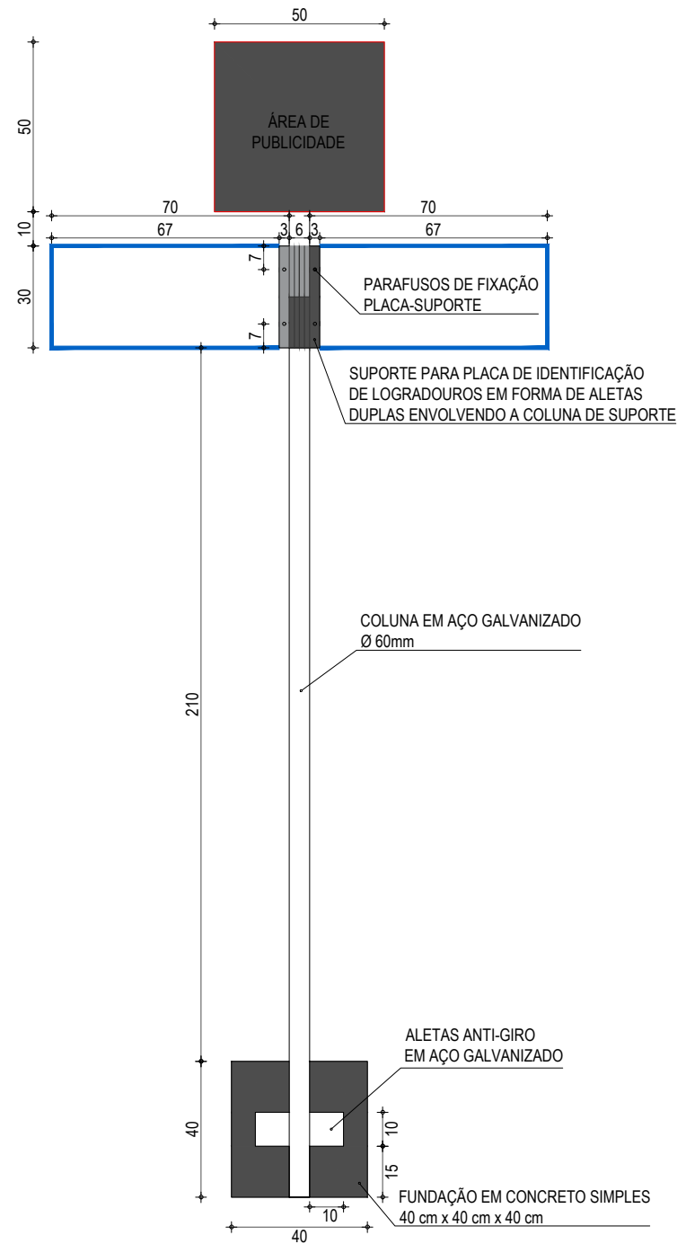
SUORTE DA PLACA ESCALA: 1/20
