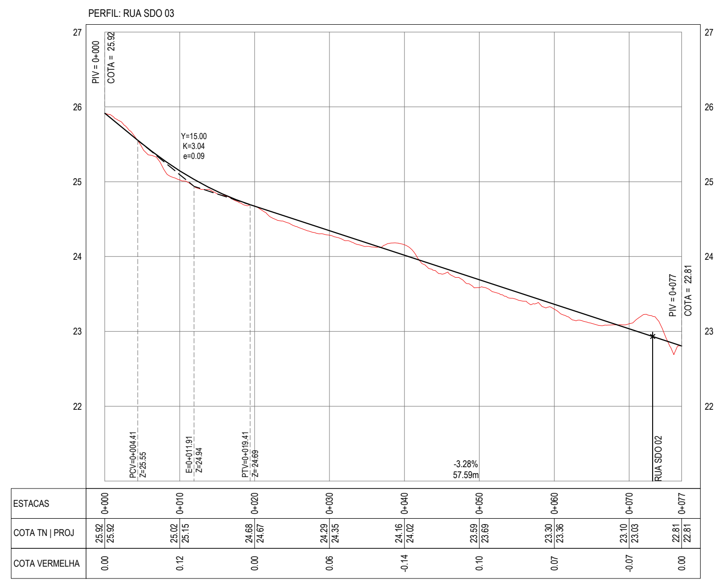
PERFIL LONGITUDINAL ESCALA: H 1/500 | V 1/50
