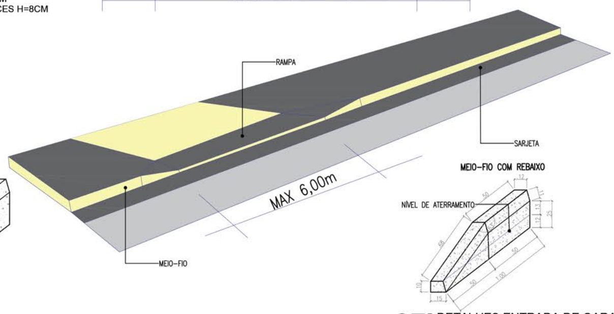
071 DETALHES ENTRADA DE GARAGENS ESCALA 1/10
