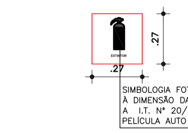
DETALHE - PLACA INDICAÇÃO EXTINTOR ESCALA 1/20
