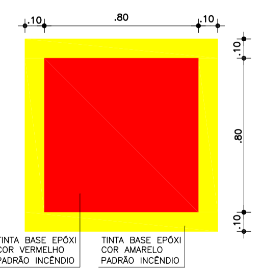
DETALHE - MARCAÇÃO PISO EXTINTOR ESCALA 1/20
