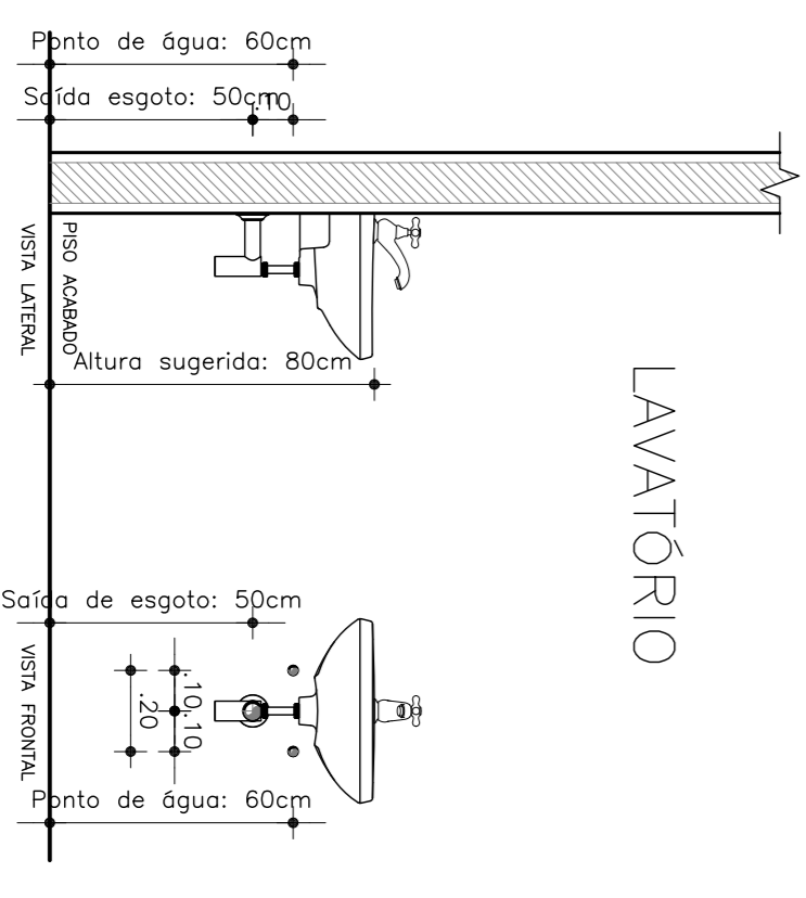
DETALHE CONSTRUTIVO ESCALA 1:20
