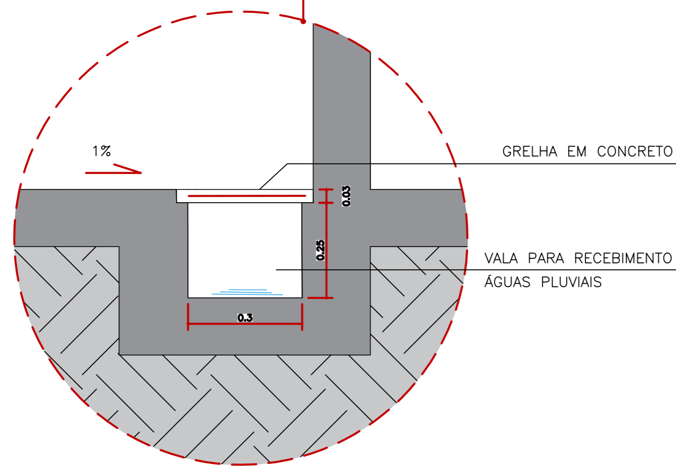
02 VALA DE DRENAGEM ESCALA 1/10
