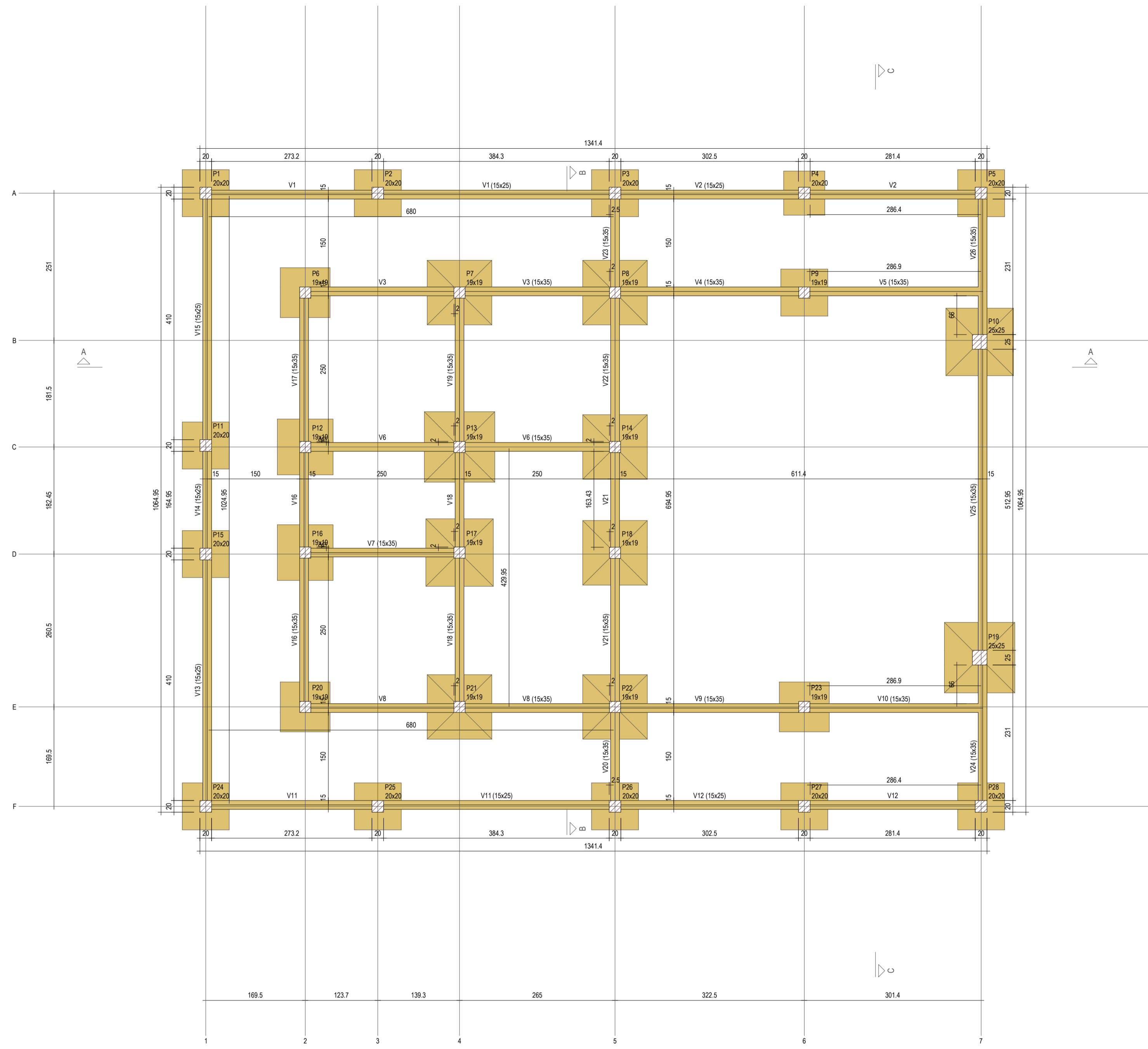
FORMA DO PAVIMENTO FUNDAÇÃO (NÍVEL 30) ESC: 1/50
