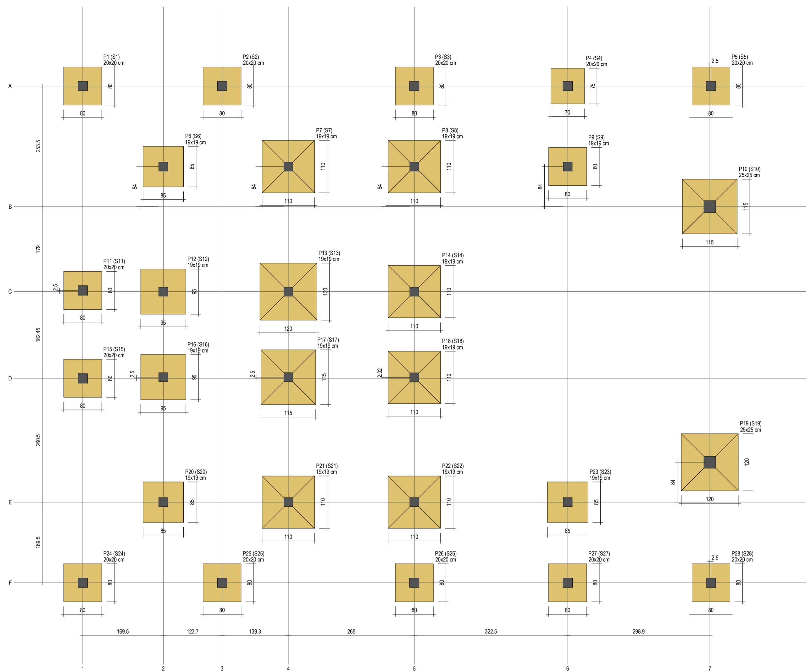
PLANTA DE LOCAÇÃO Esc. 1:50
