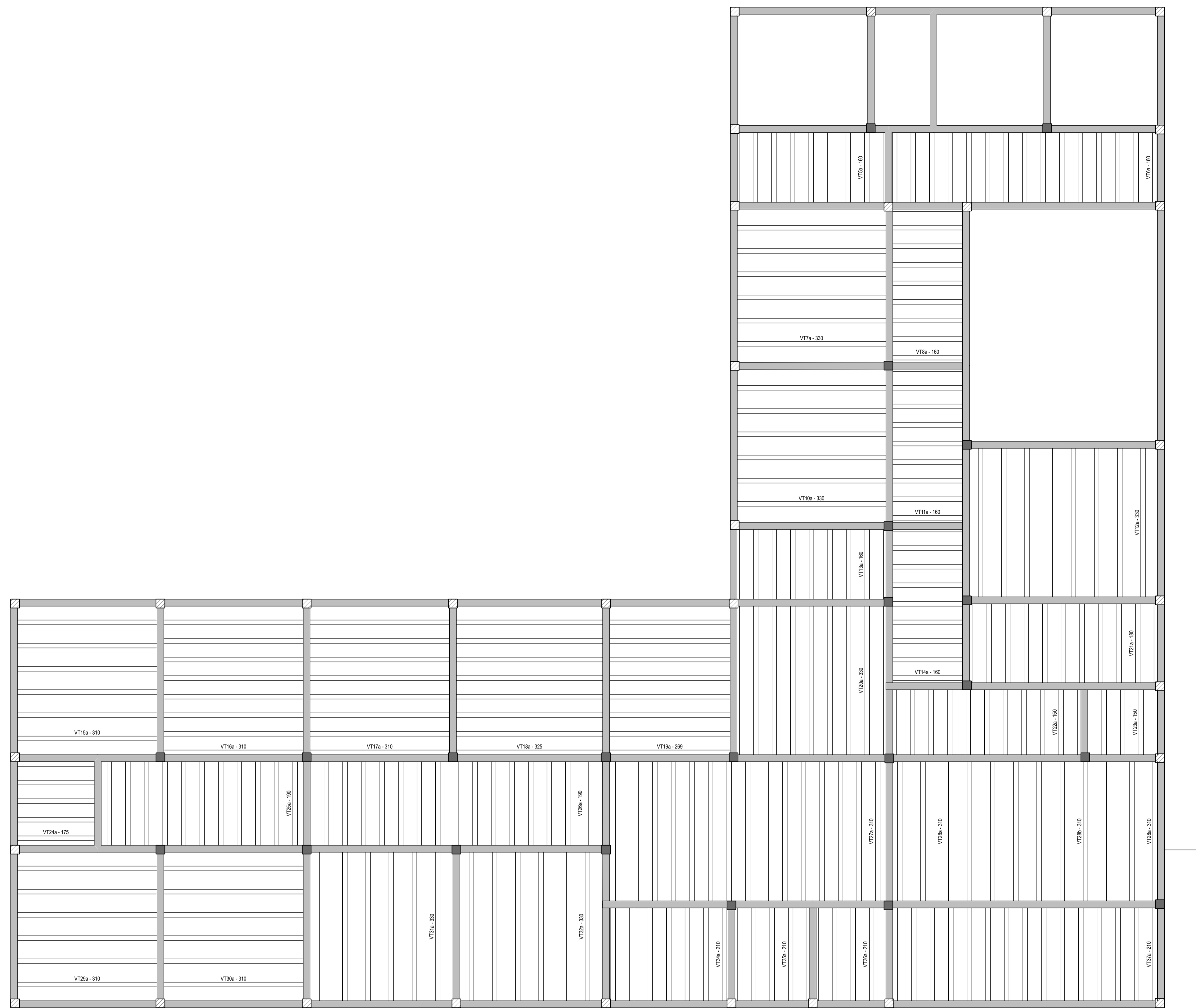
PLANTA DE VIGOTAS PRÉ-MOLDADAS ESC. 1/50
