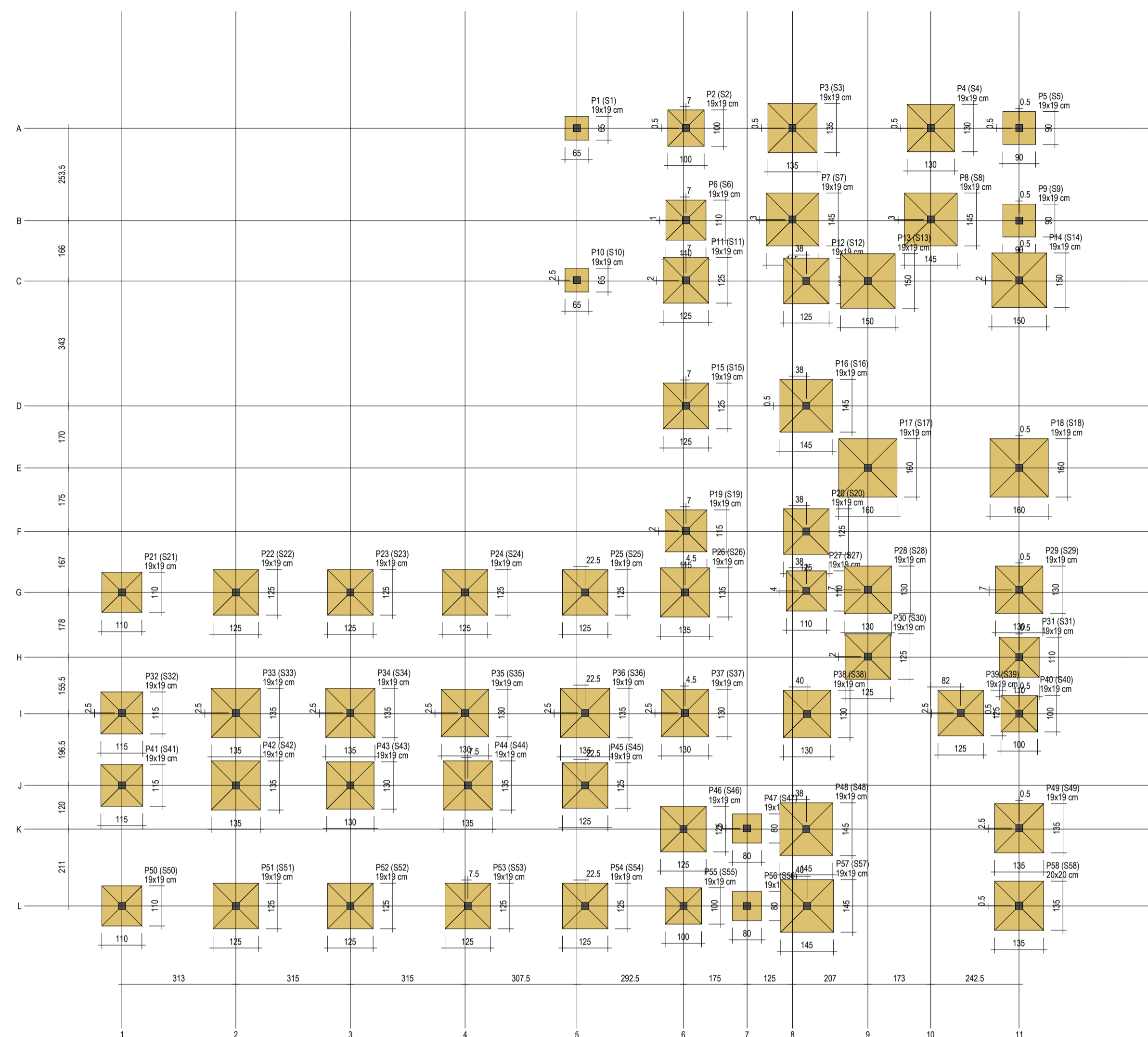
PLANTA DE LOCAÇÃO ESC. 1:100
