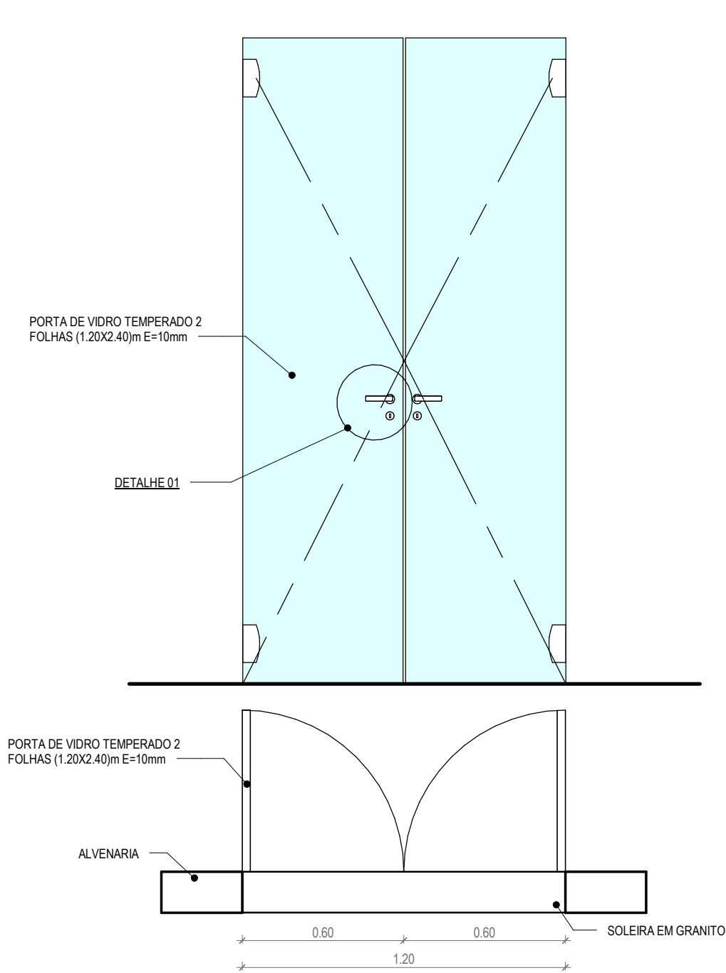
4 | PORTA DE ALUMÍNIO E VIDRO - P04 1:20
