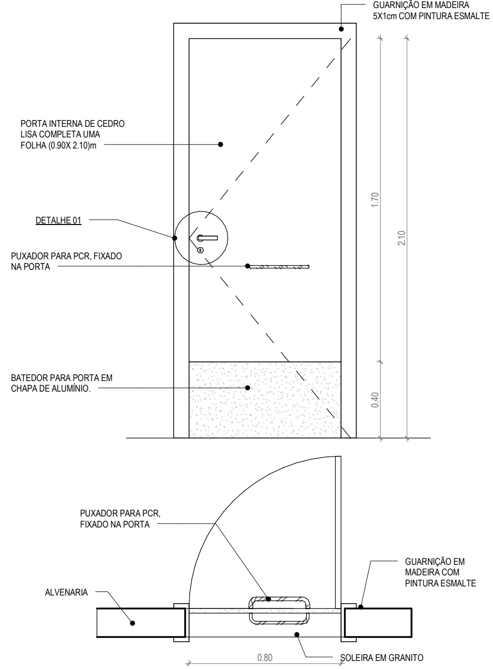
2 | PORTA PADRÃO - P02 1:20
