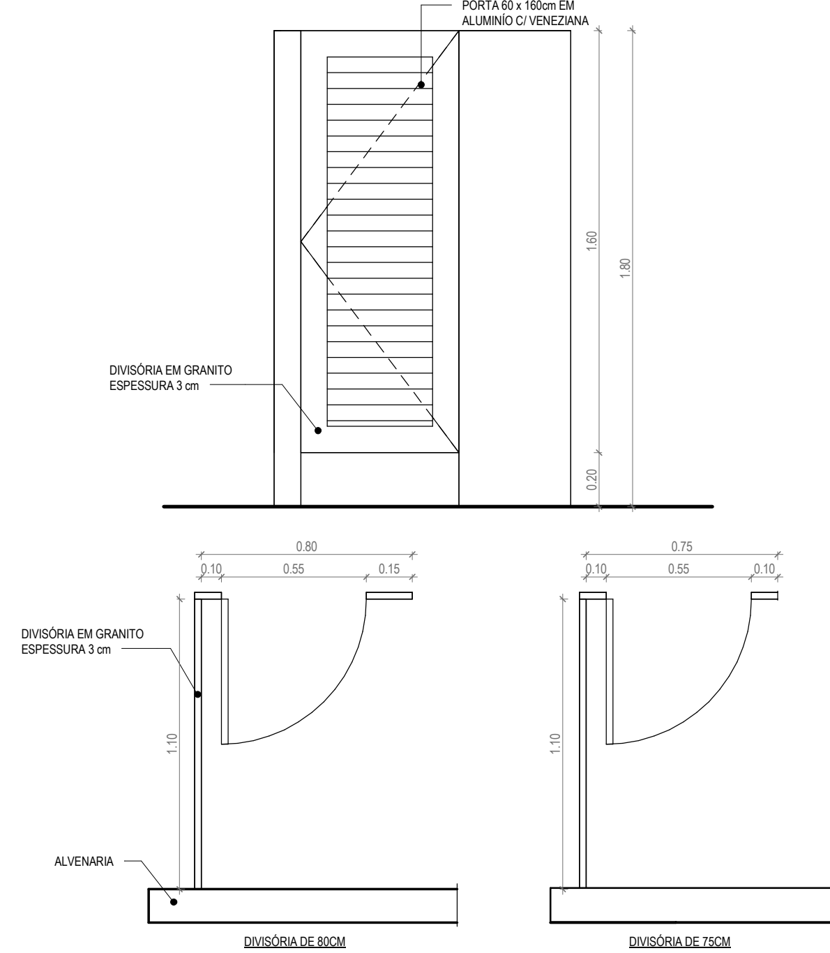
3 | PORTA DE ALUMÍNIO - P03 1:20
