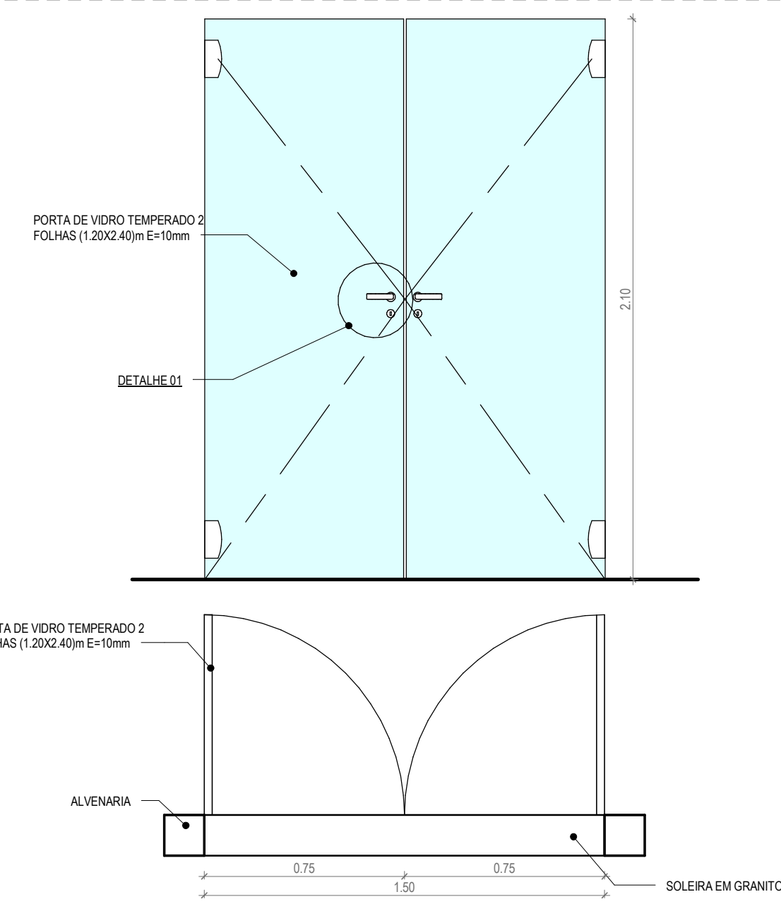
1 | PORTA PADRÃO - P01 1:20
