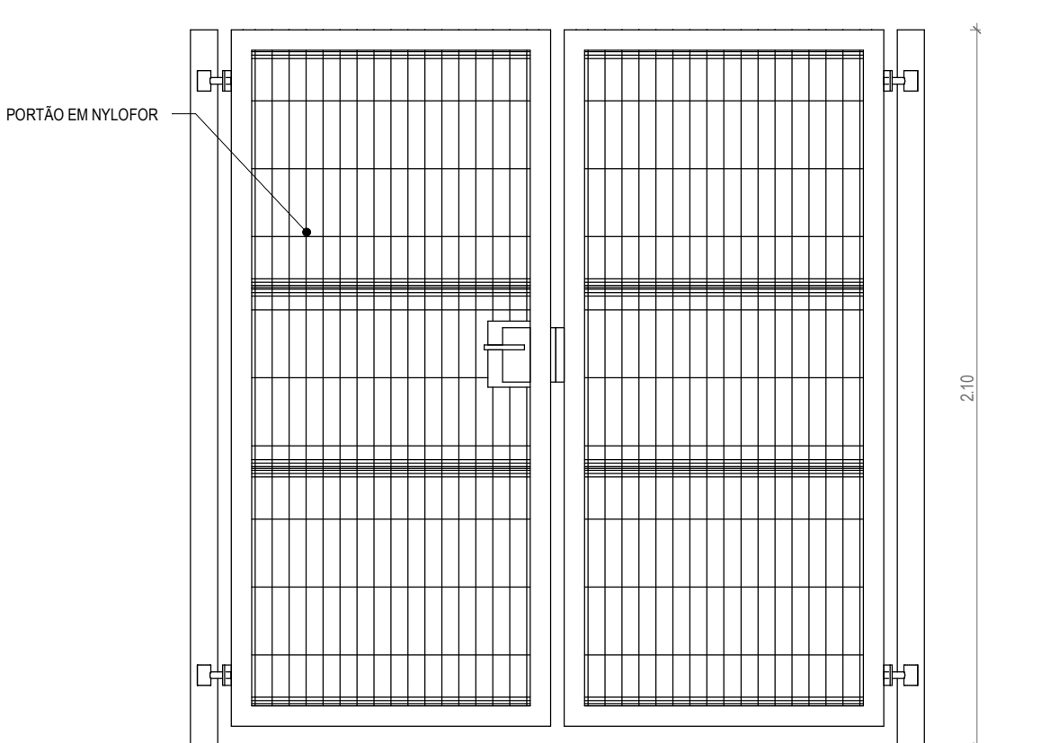
10 | PORTÃO DE NYLÓFOR - P10 1:20
