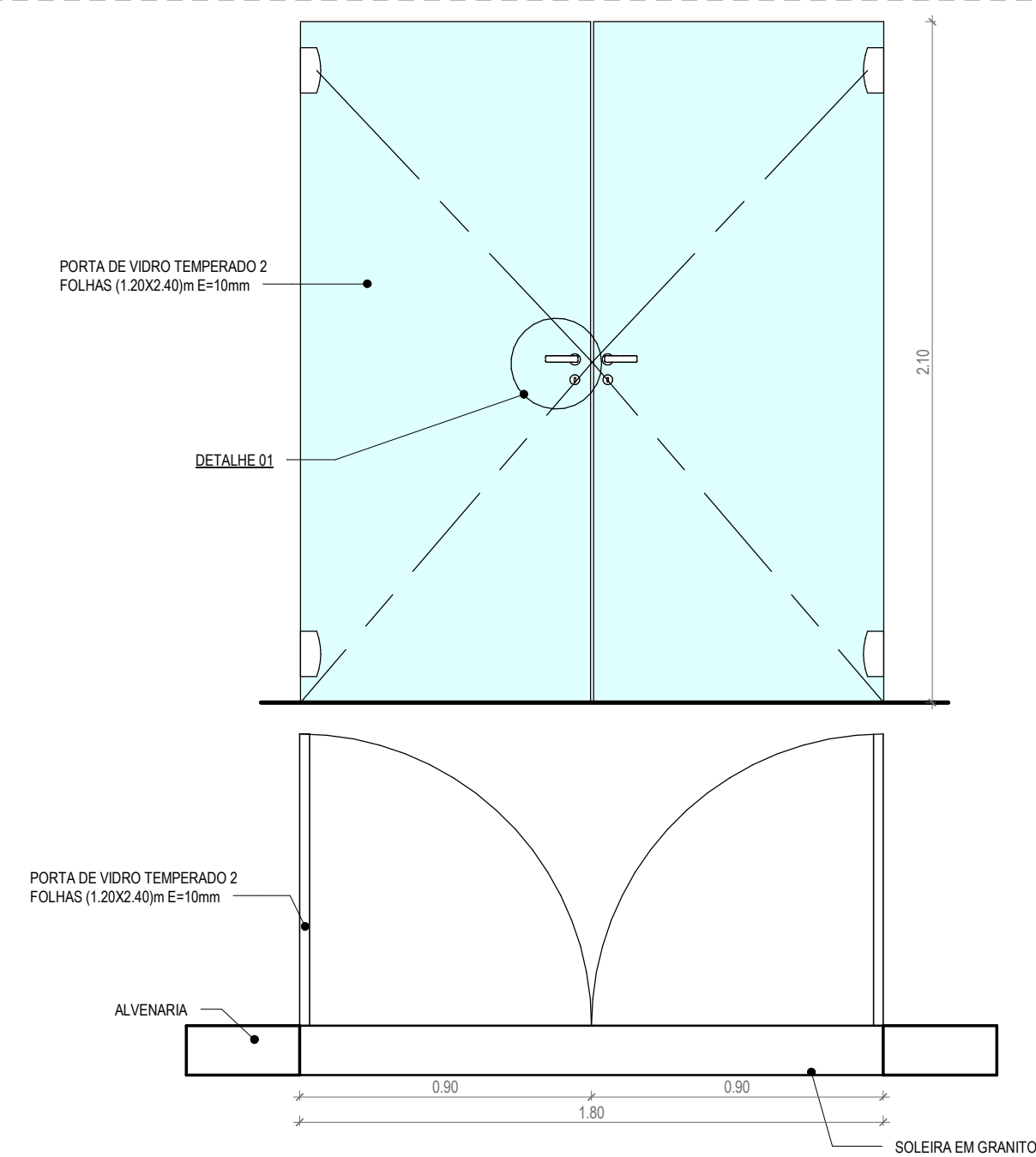
6 | PORTA DE ALUMÍNIO E VIDRO - P06 1:20
