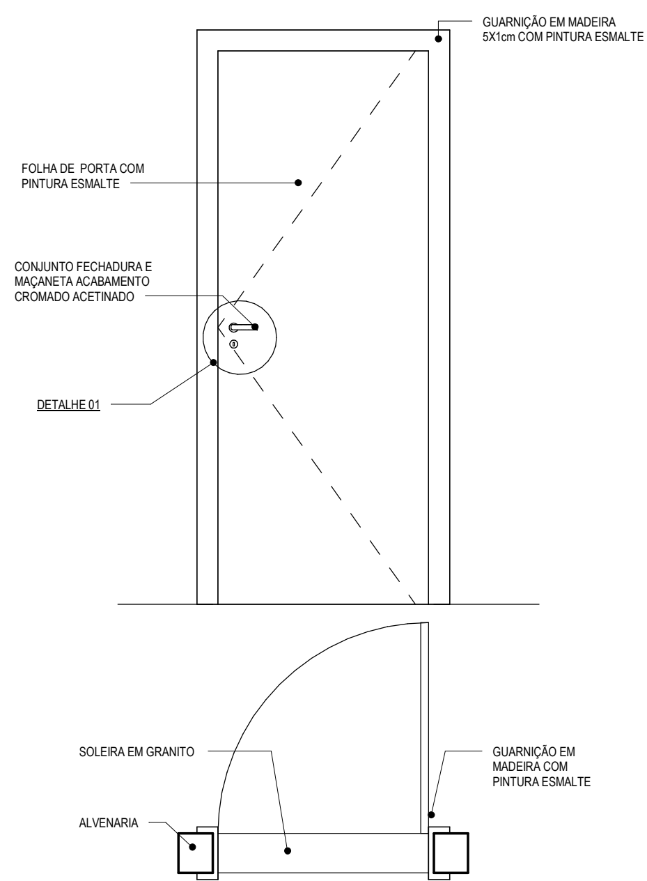
1 | PORTA PADRÃO - P01 1:20
