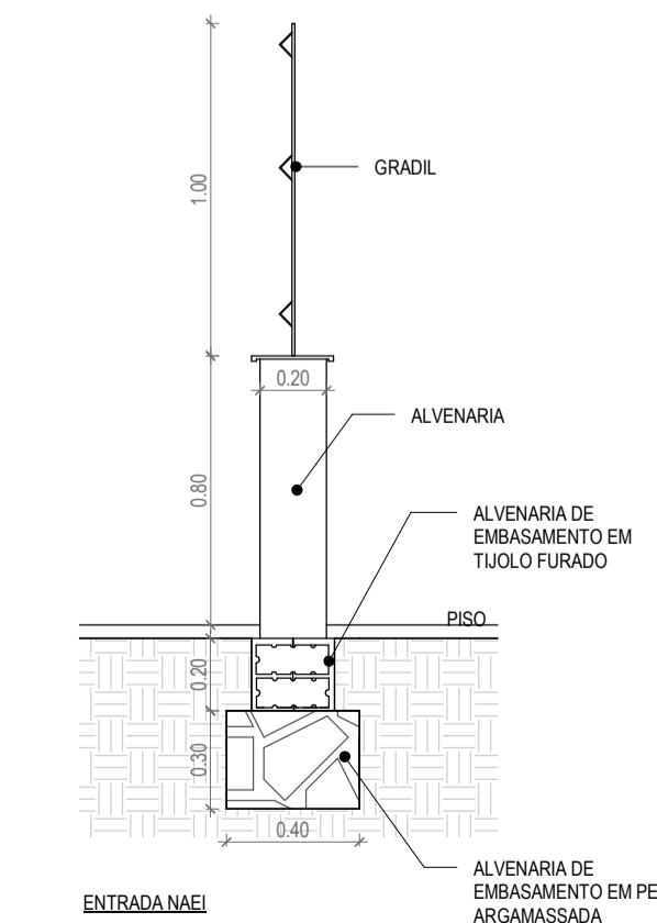
6 DETALHE DA MURETA E GRADIL 1:25
