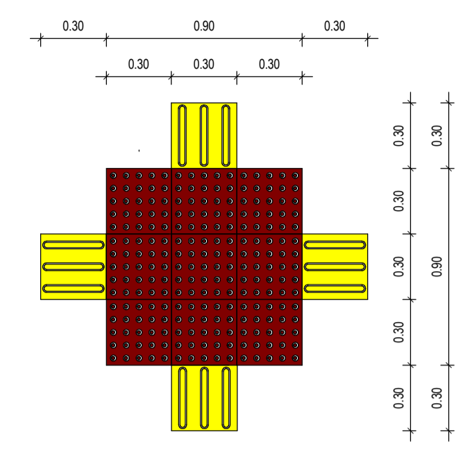
2 | DET. ENCONTRO PISO PODOTÁTIL INTERNO 4 DIREÇÕES 1:20
