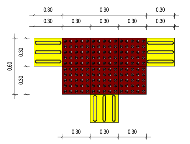
4 | DETALHE ENCONTRO PISO PODOTÁTIL INTERNO 3 DIREÇÕES 1:20
