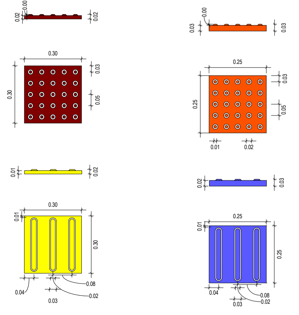
6 | DET. PODOTÁTIL INTERNO 1:10
