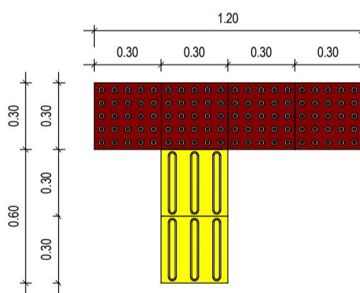
5 | DETALHE ENCONTRO PISO PODOTÁTIL INTERNO 1 DIREÇÃO 1:20
