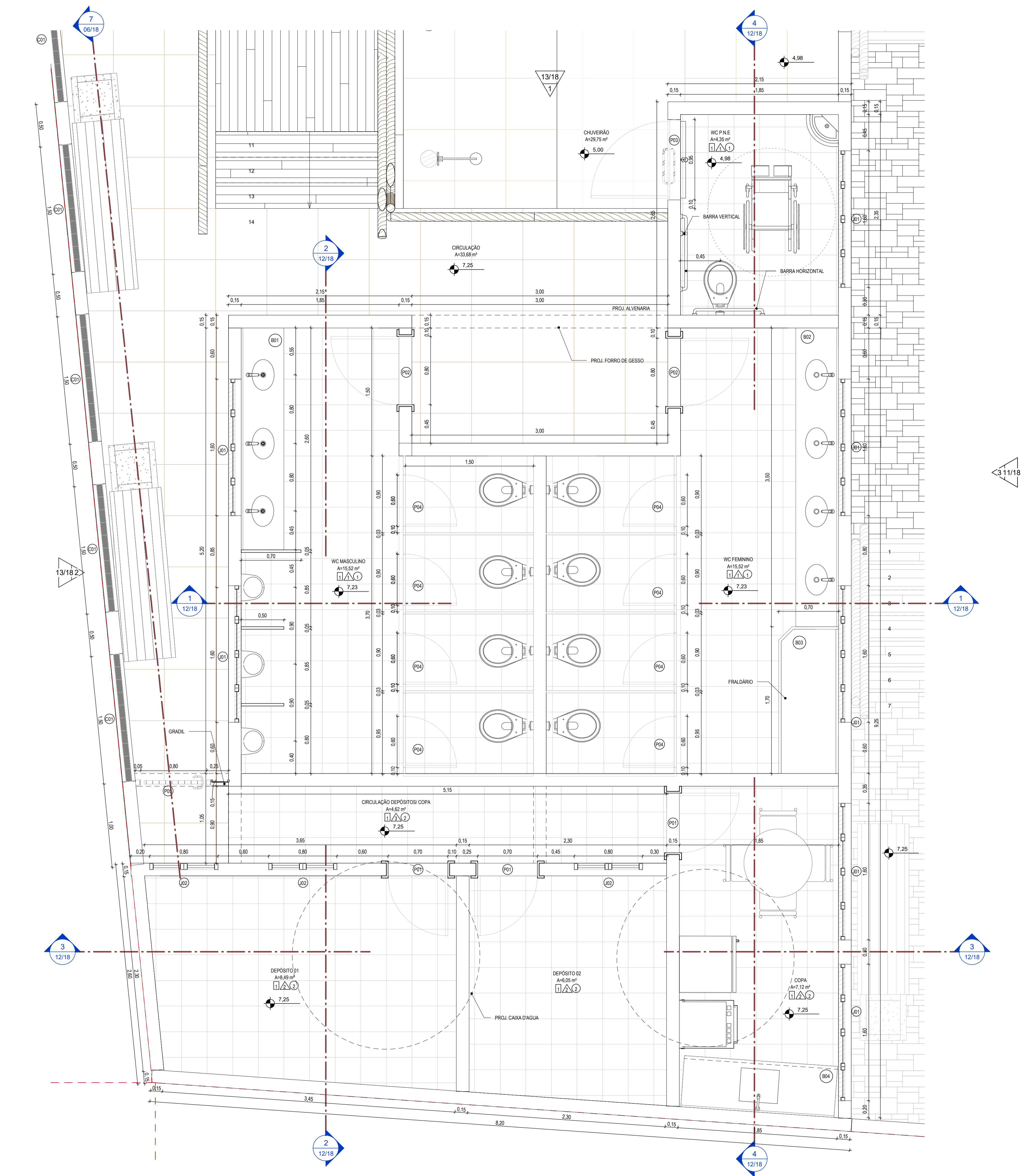
1 PLANTA BAIXA - VESTIÁRIOS E DEPÓSITO 1:25
