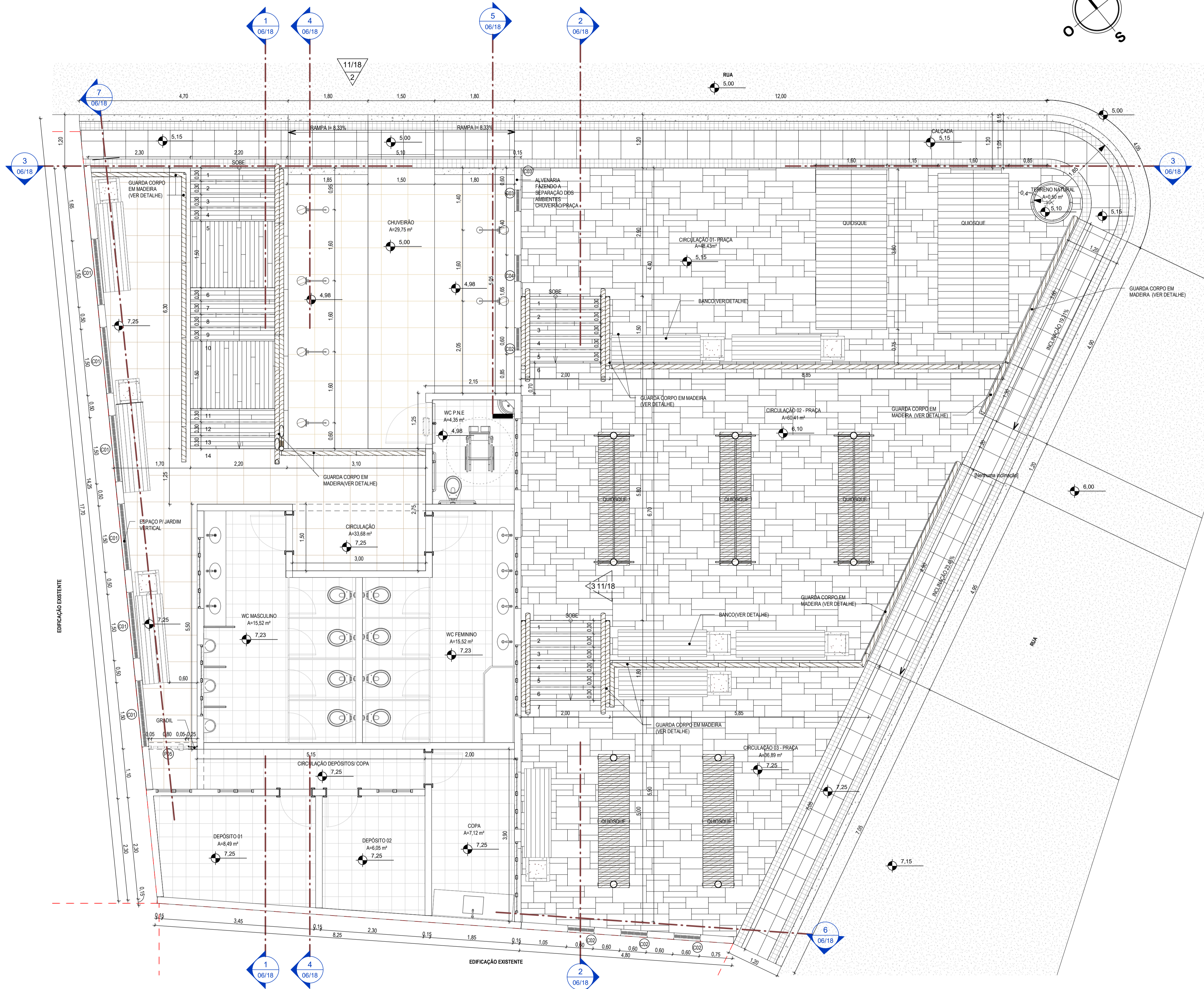
1 PLANTA TÉCNICA - CHUVEIRÃO 1:50
