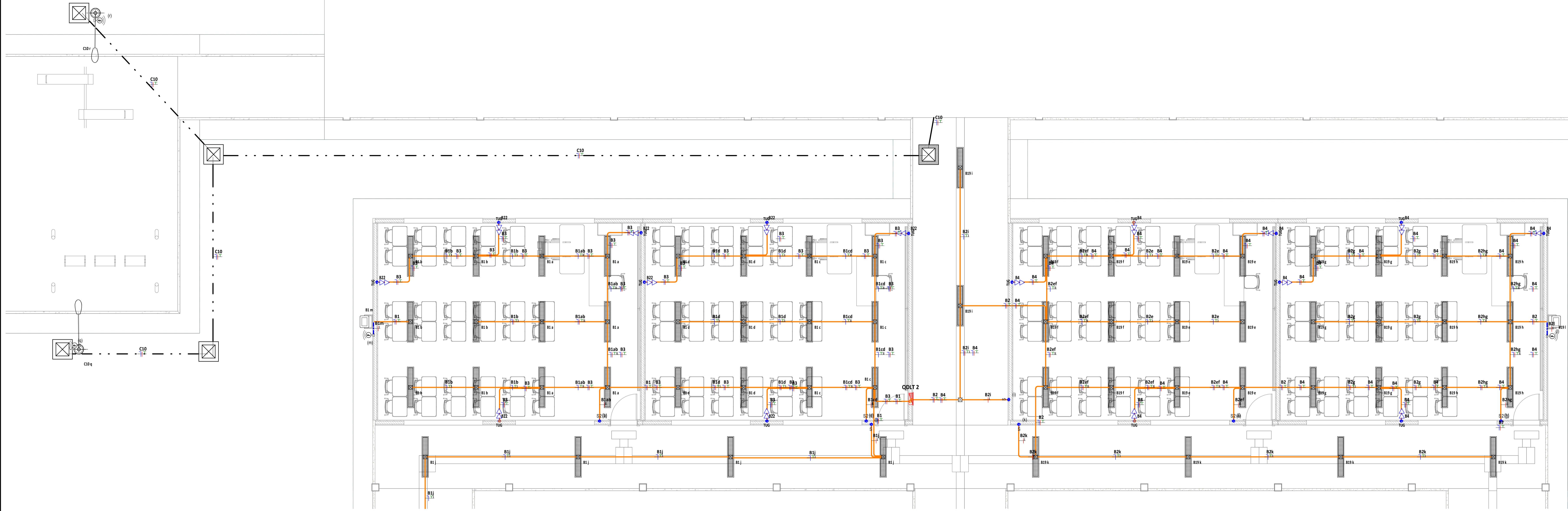
LUM E TOMADAS - BLOCO 2 1:50
