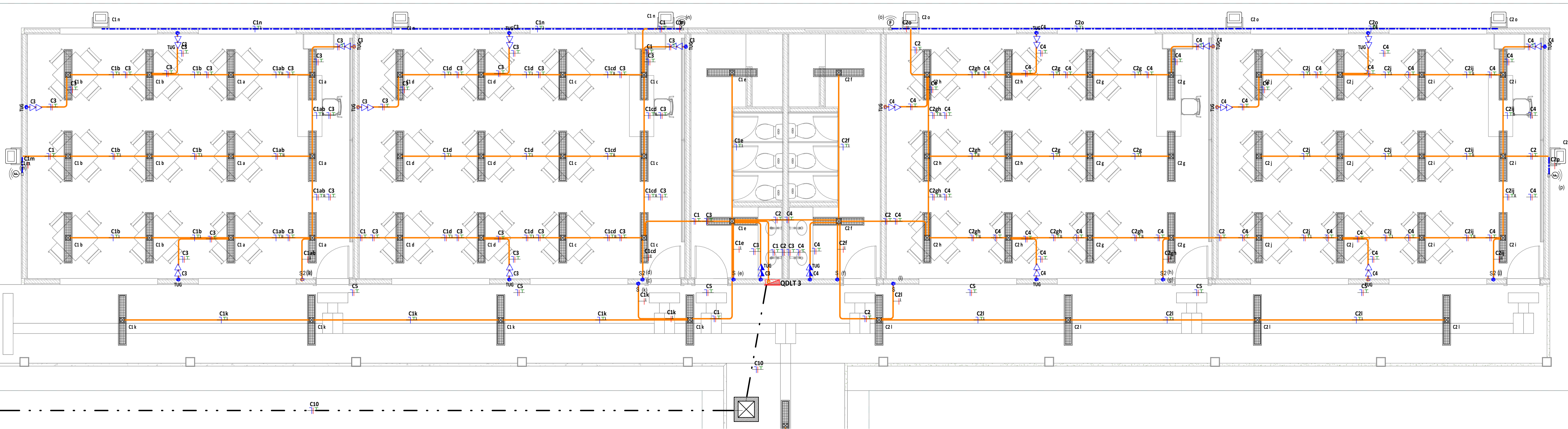
LUM E TOMADAS - BLOCO 3 1:50
