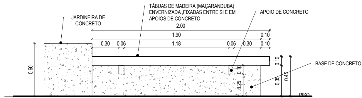
VISTA
