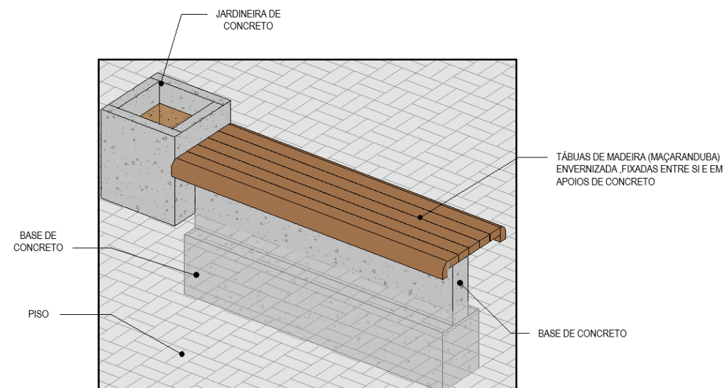
PERSPECTIVA
