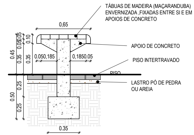
CORTE BANCO
