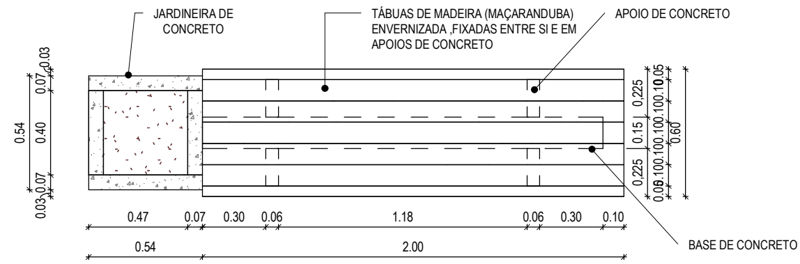
PLANTA
