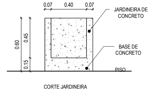
CORTE JARDINEIRA
