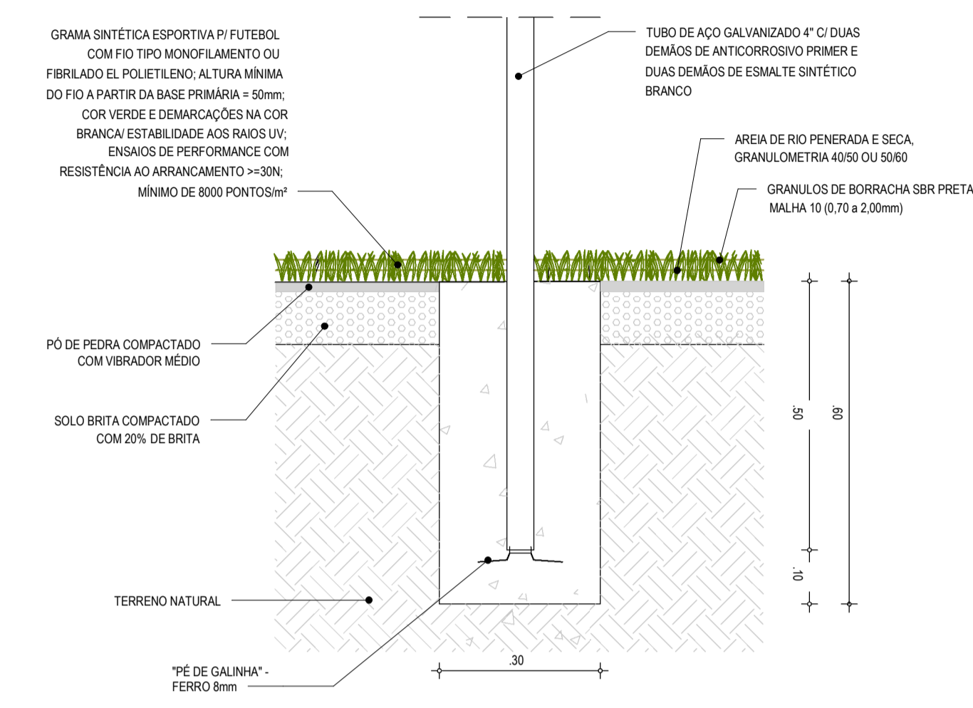
4 DETALHE - CHUMBAMENTO DA TRAVE 1:10
