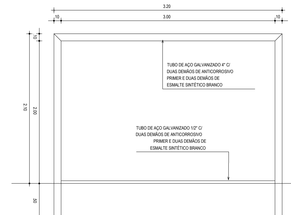
3 VISTA FRONTAL - TRAVE 1:25
