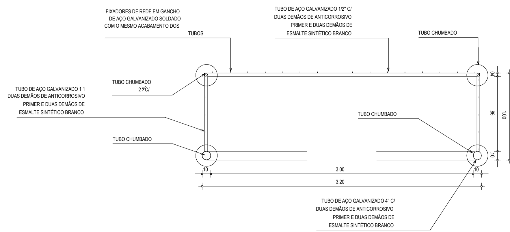
1 PLANTA BAIXA - TRAVE 1:25
