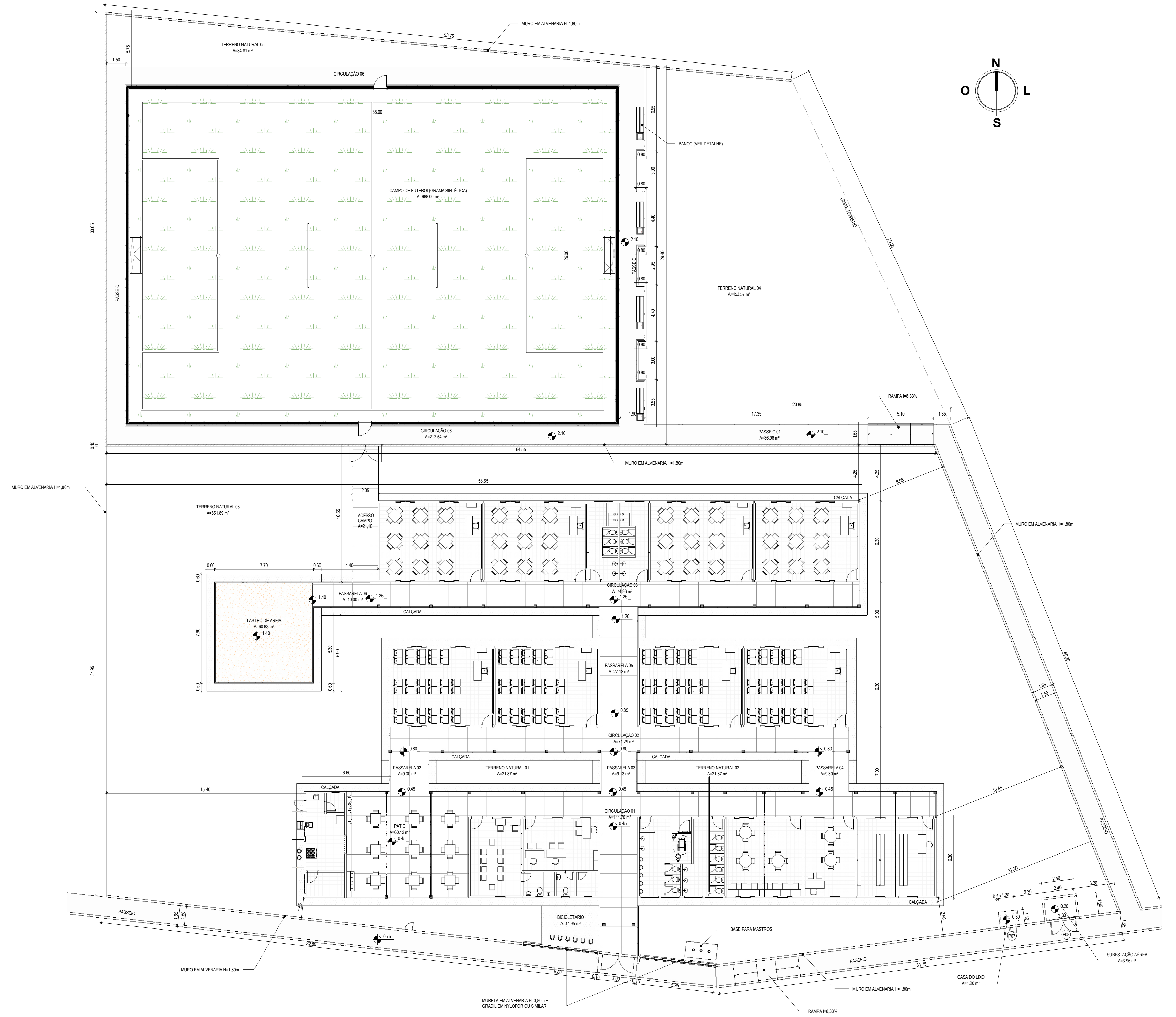
1 PLANTA BAIXA GERAL 1 : 150
