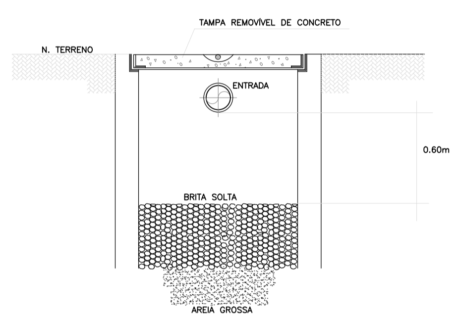
04 DETALHE DA CAIXA DE ÁREA ESC.: 1/100
