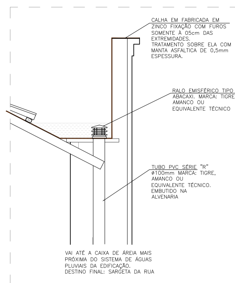
03 DETALHE GÊNÉRICO DA CALHA ESC.: 1/100
