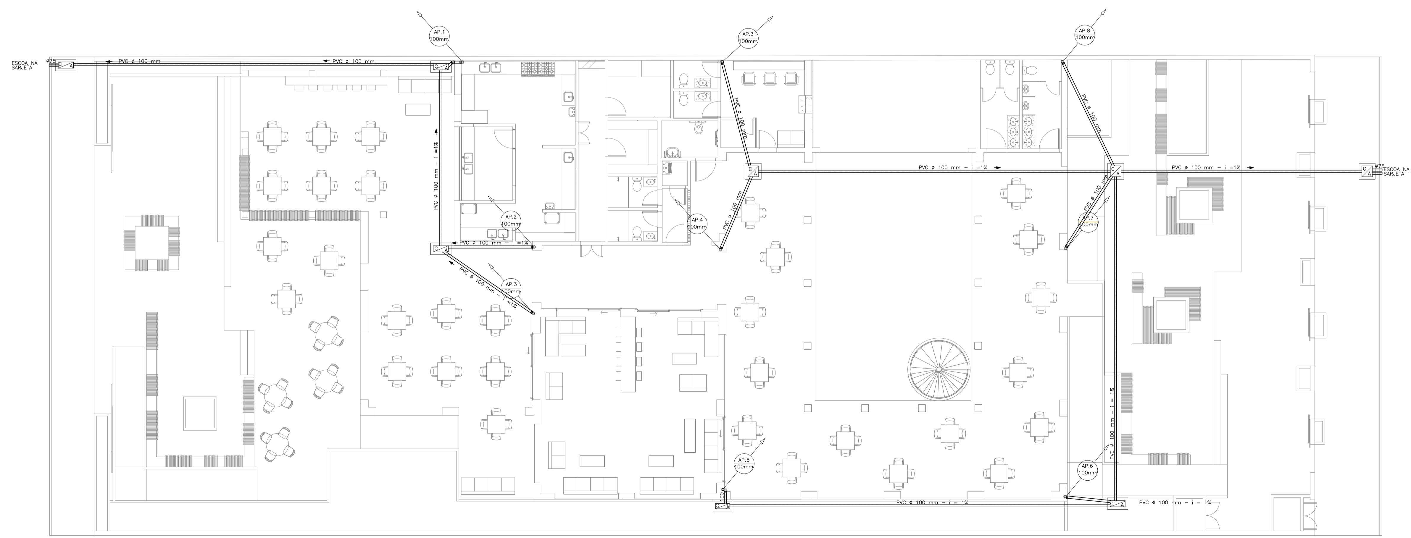
02 PLANTA TÉRREO ESC.: 1/100
