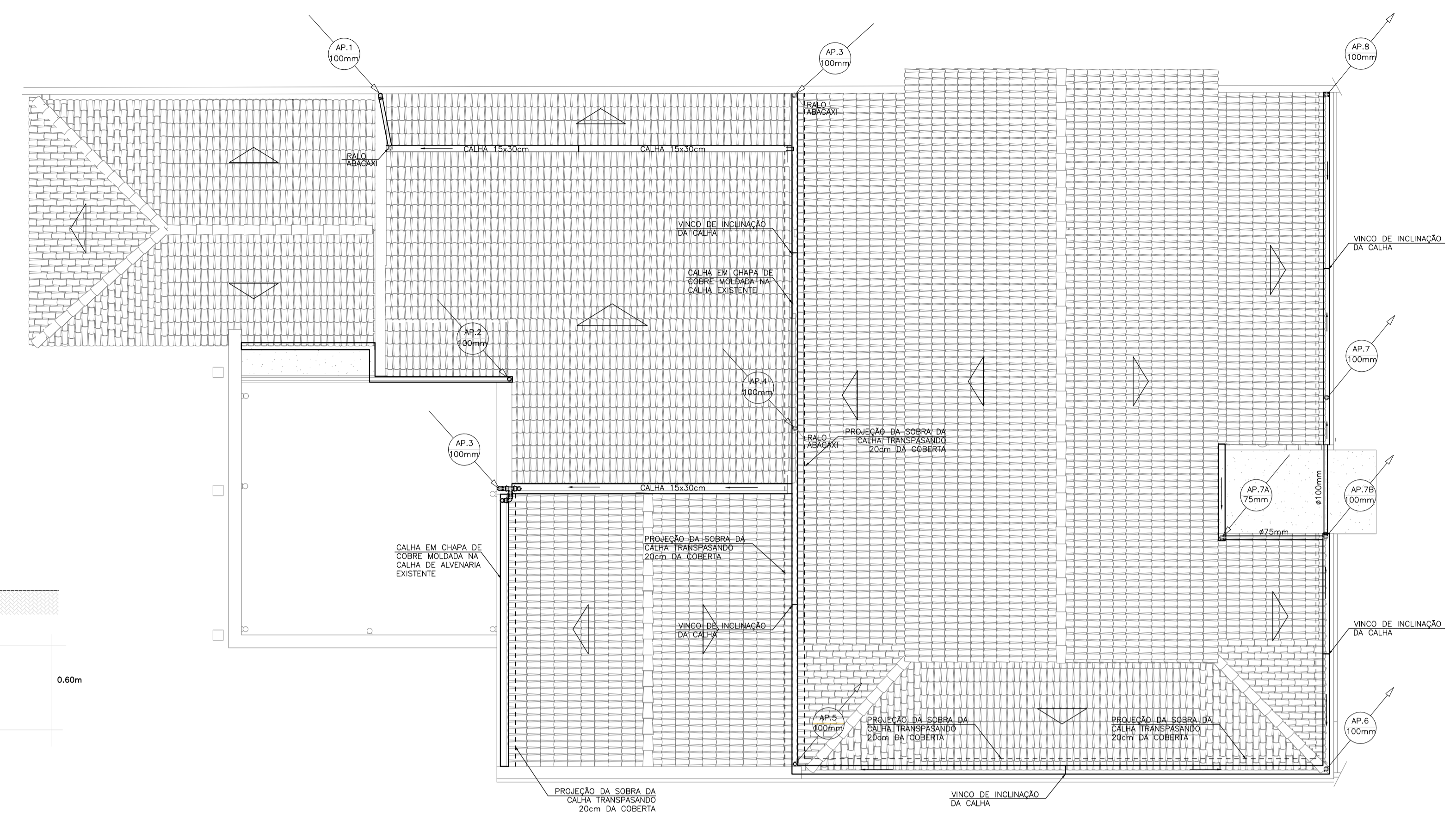
01 PLANTA DE COBERTA ESC.: 1/100
