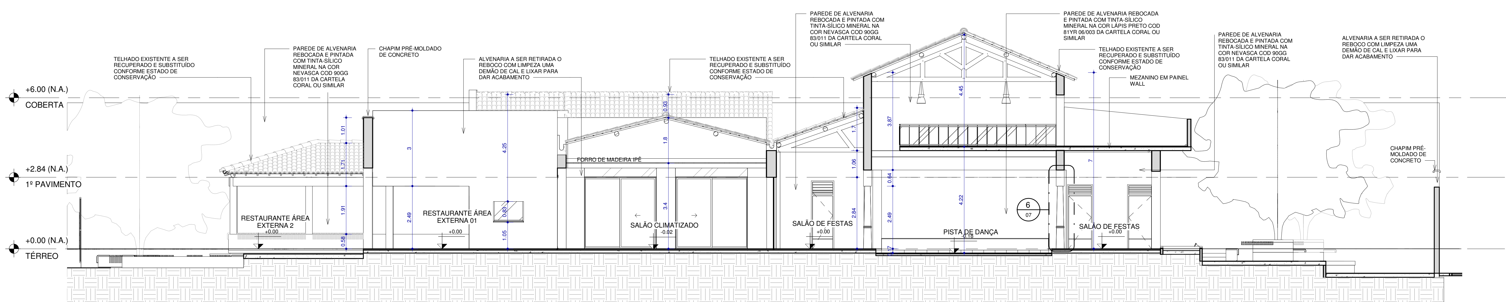
3 CORTE 1 CONSTRUÇÃO 1:75
