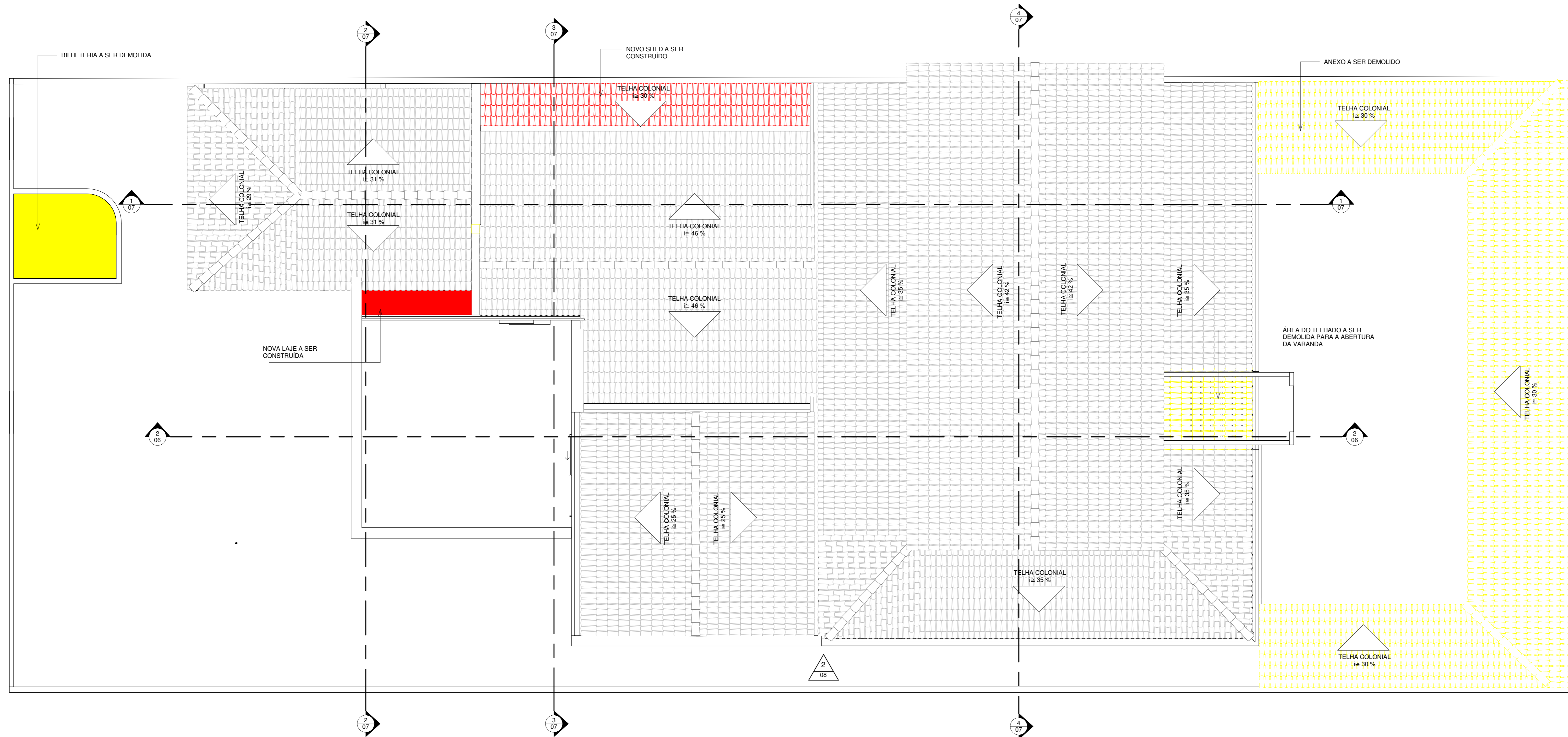
1 PLANTA DE DEMOLIR/CONSTRUIR 1 : 75
