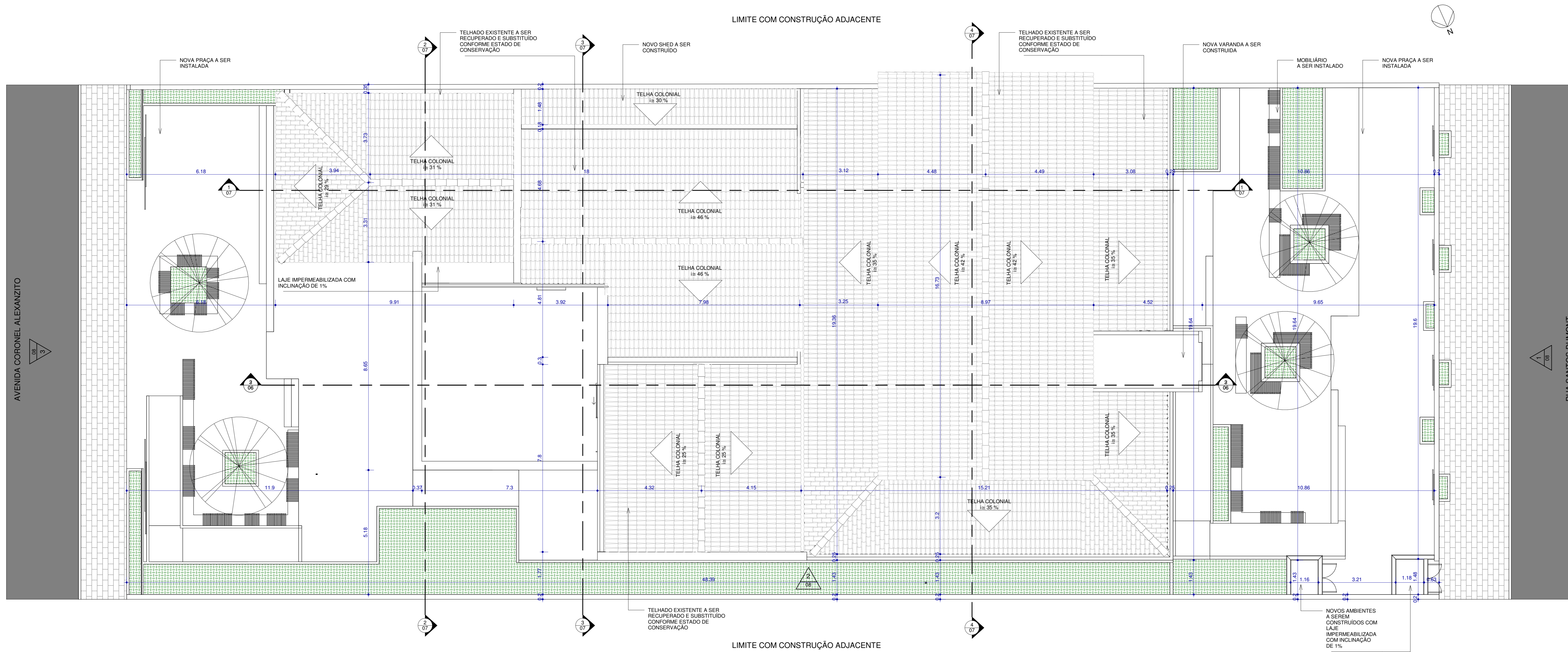
1 PLANTA DE SITUAÇÃO E COBERTA 1 : 75
