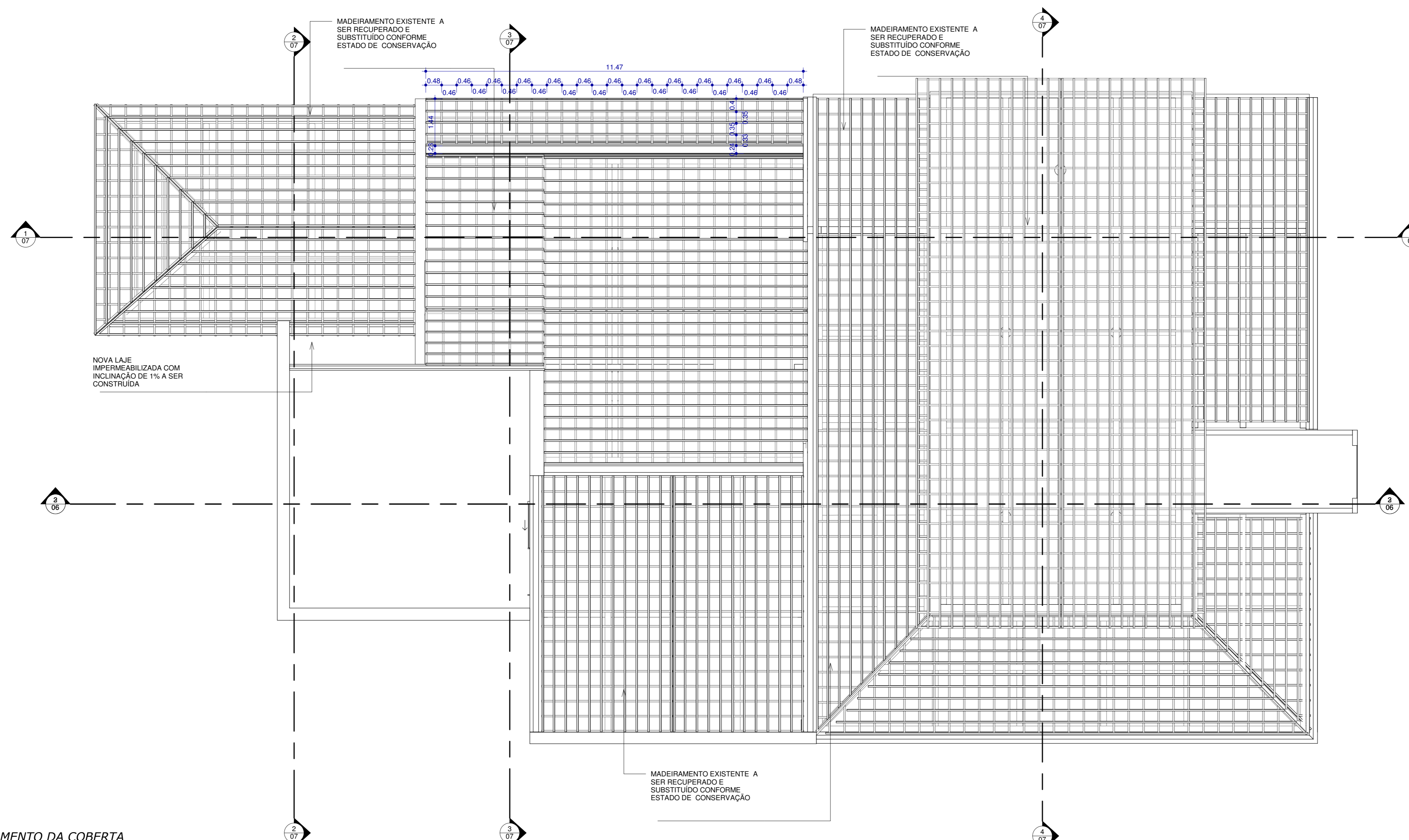
2 PLANTA DE MADEIRAMENTO DA COBERTA 1 : 75
