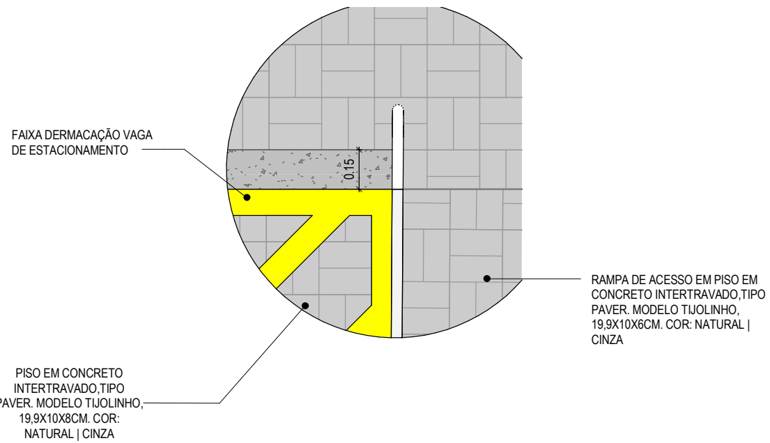
2 | DETALHE 01 1:20
