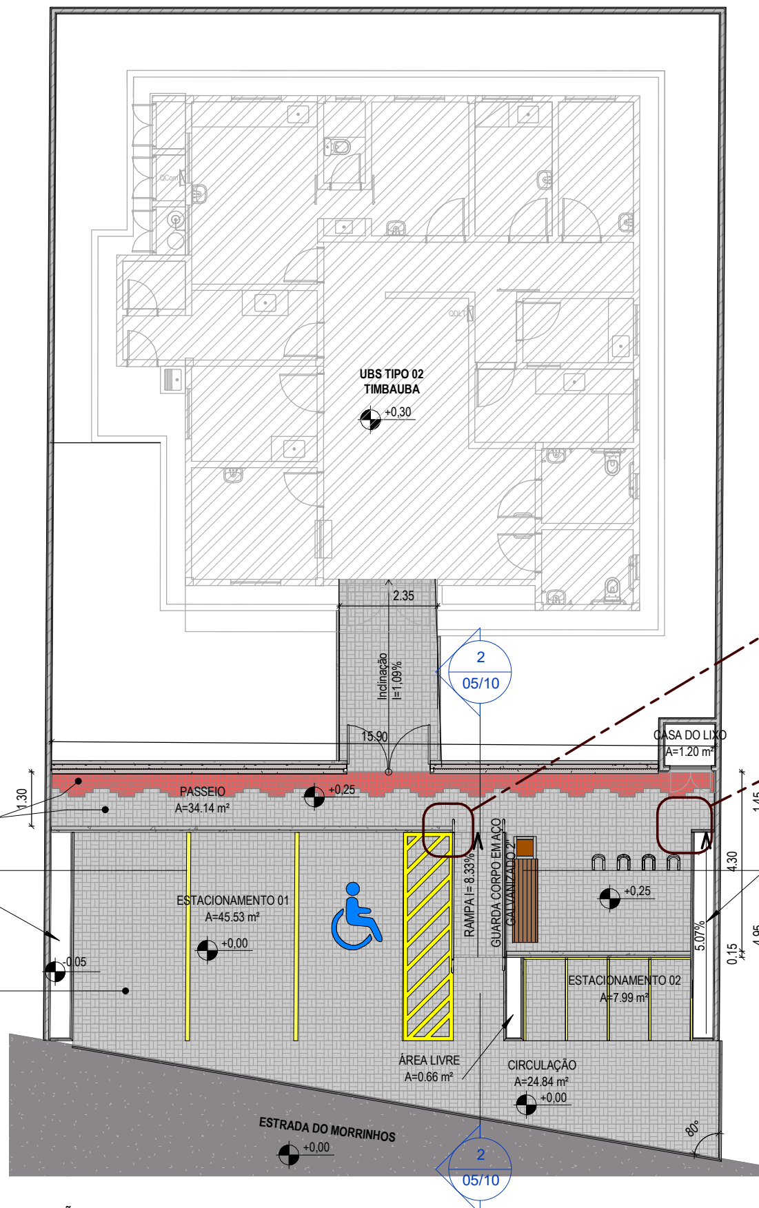
1 | PLANTA PAGINAÇÃO DE PISO - TIMBAUBA 1 : 125
