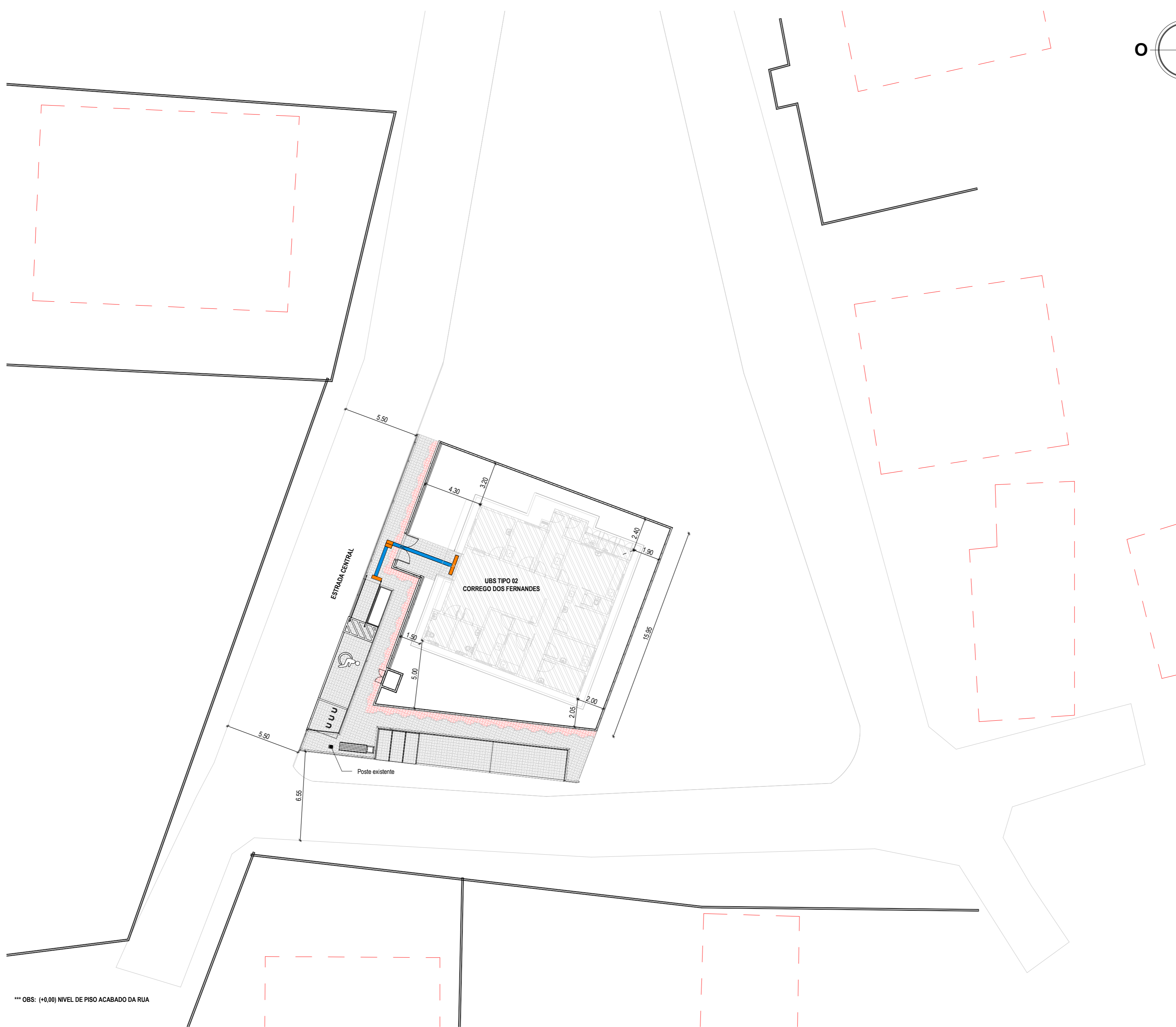
1 PLANTA DE LOCAÇÃO - UBS CORREGO DOS FERNANDES 1 : 200
