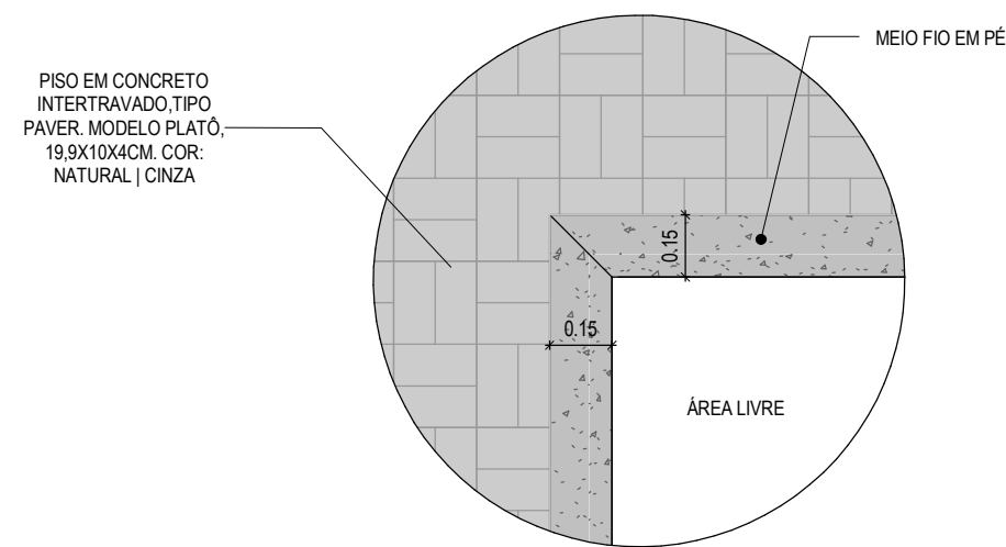
2 | DETALHE 01 1:20
