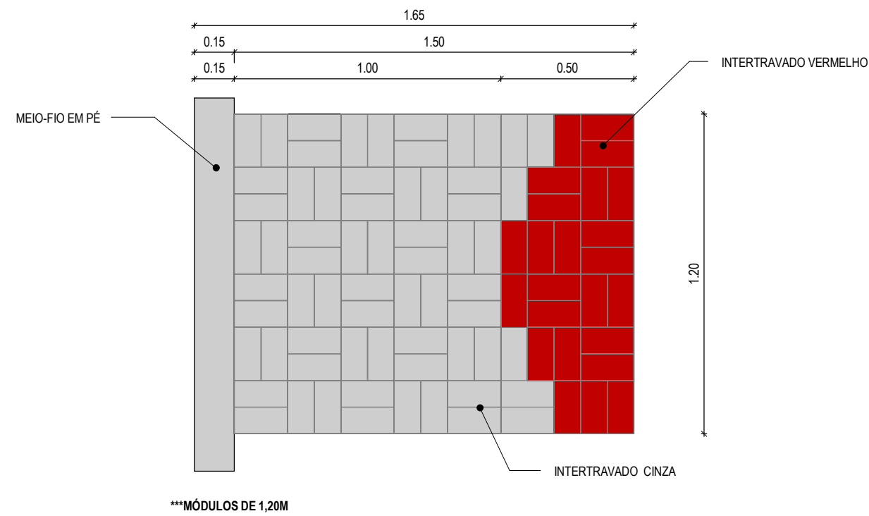
1 | DETALHE 01 - PAGINAÇÃO DE PISO EXTERNO 1:20
