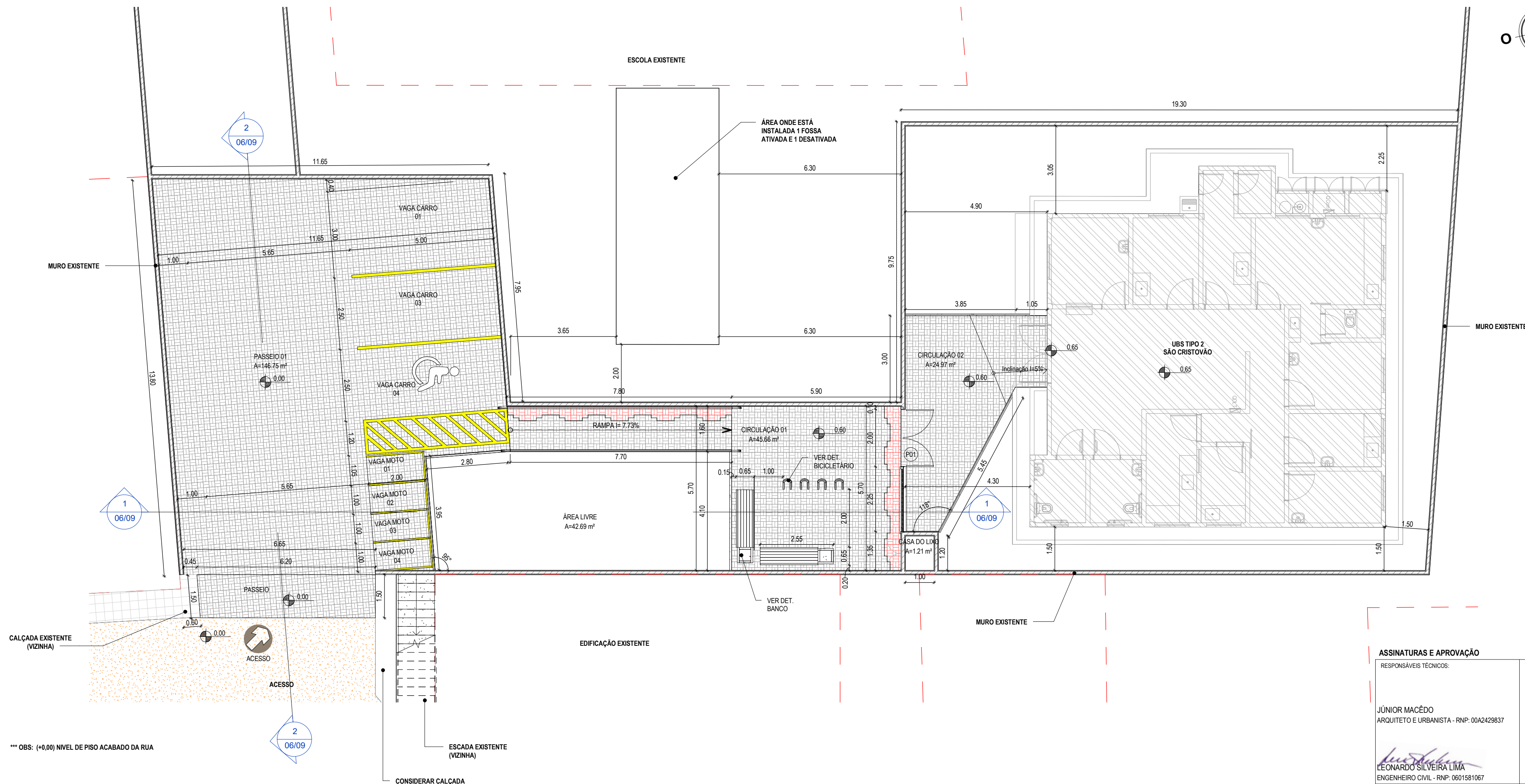
1 | PLANTA TÉCNICA 1:100
