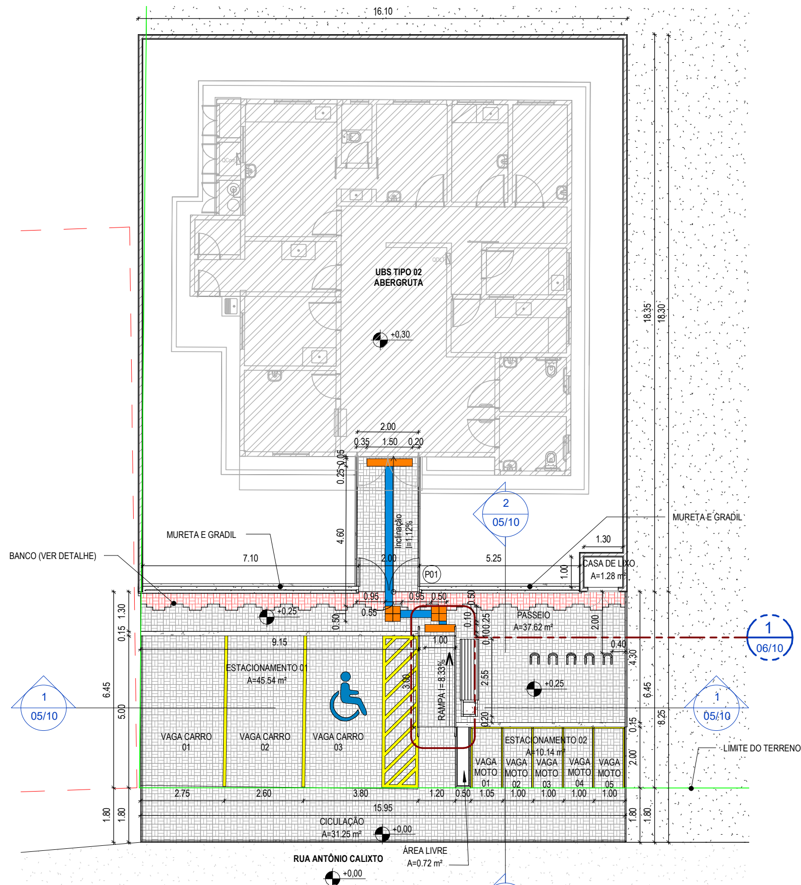
1 PLANTA TÉCNICA - ABERGRUTA 1: 125
