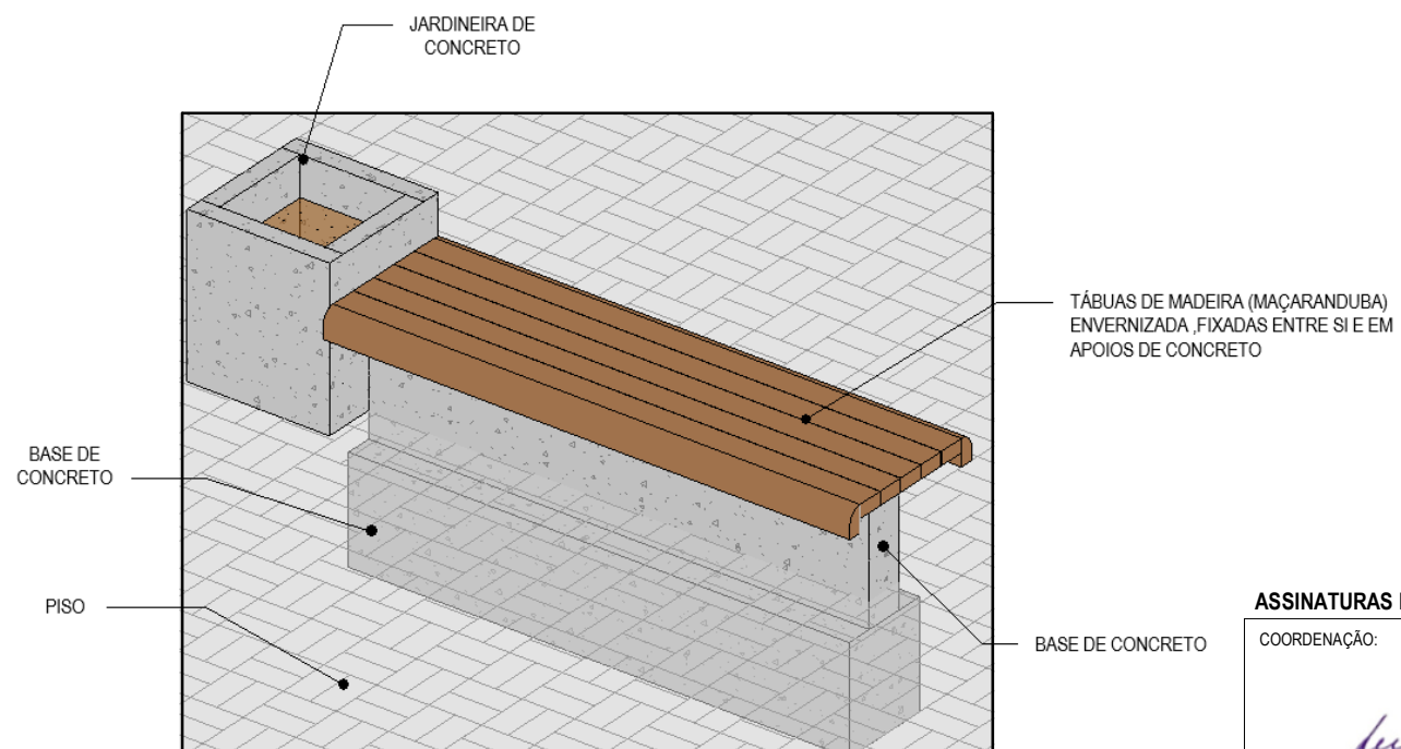
DETALHE BANCO 1 : 20
