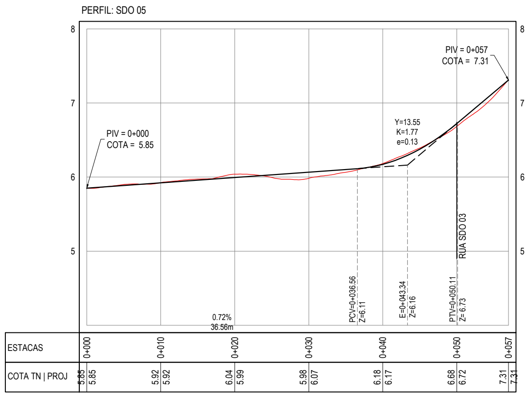
PERFIL LONGITUDINAL ESCALA: H 1/500 | V 1/50
