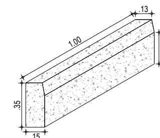
DETALHE DO MEIO FIO ESCALA: 1/30
