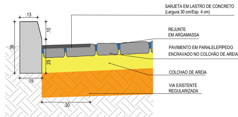
DETALHE DOS MATERIAIS ESCALA: SEM ESCALA
