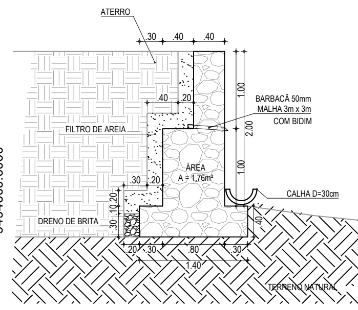
② DETALHE DO MURO DE ARRIMO esc.: 1/50
