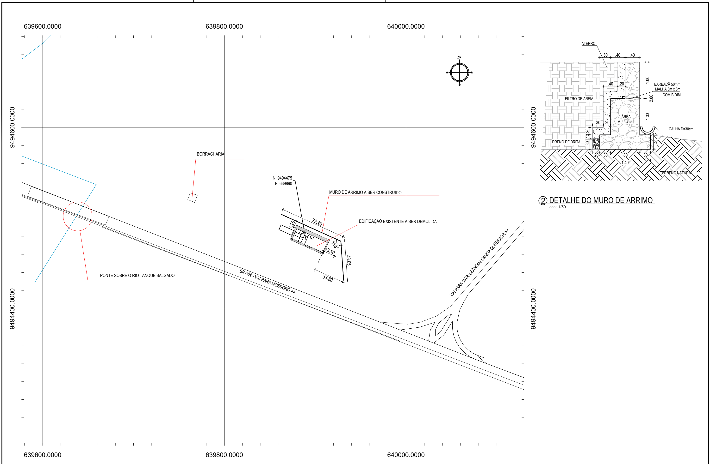
① PLANTA DE LOCALIZAÇÃO esc.: 1/2.000
