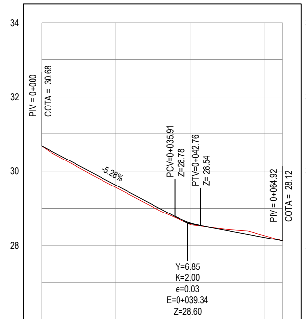
PERFIL: RUA ARMANDO ROCHA 06
