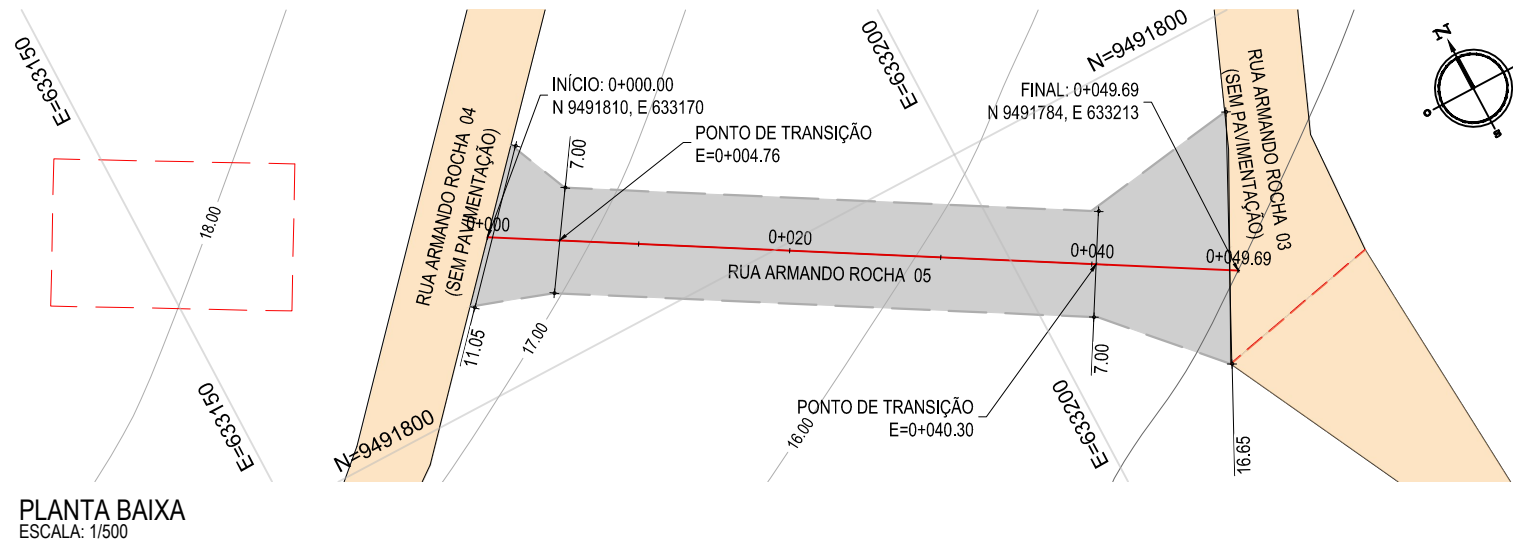
PERFIL: RUA ARMANDO ROCHA 05
