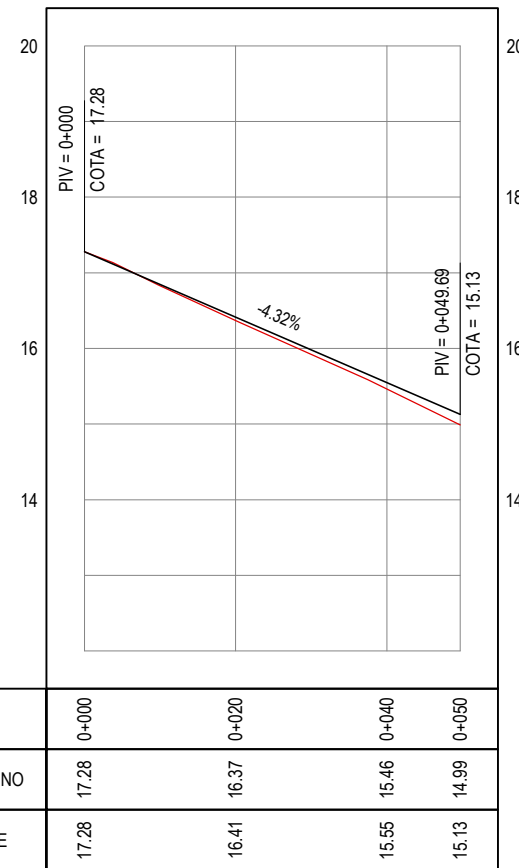
PERFIL LONGITUDINAL ESCALA: H 1/1000 | V 1/100
