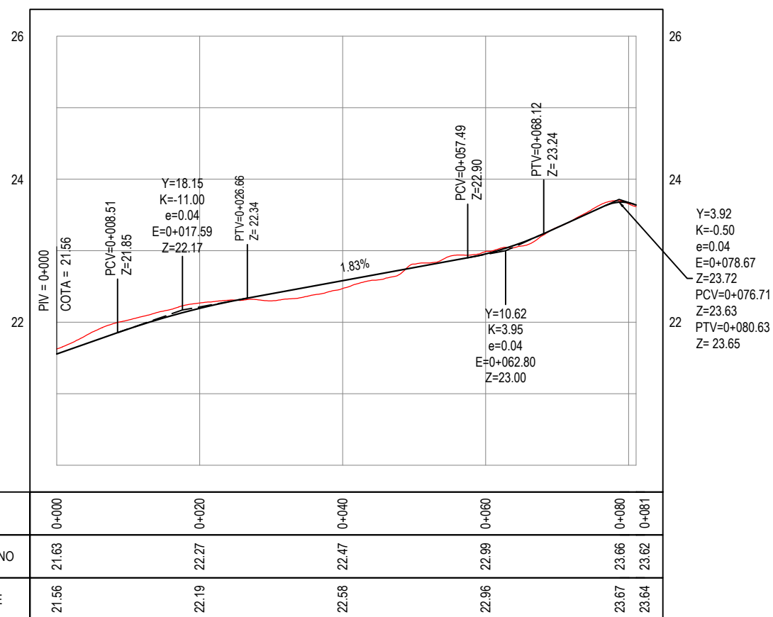
PERFIL LONGITUDINAL ESCALA: H 1/750 | V 1/75
