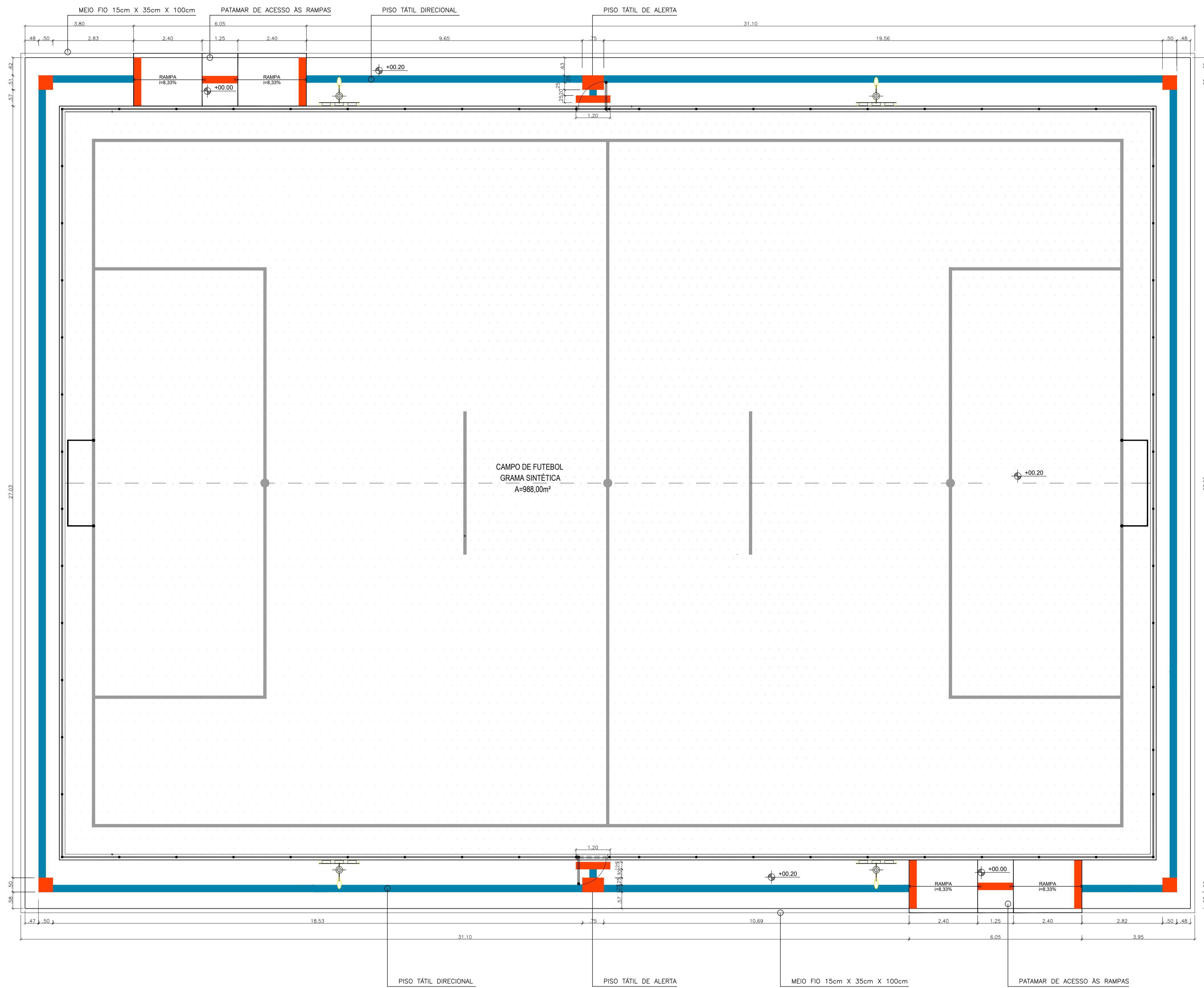
01 PLANTA ACESSIBILIDADE ESCALA 1/75
