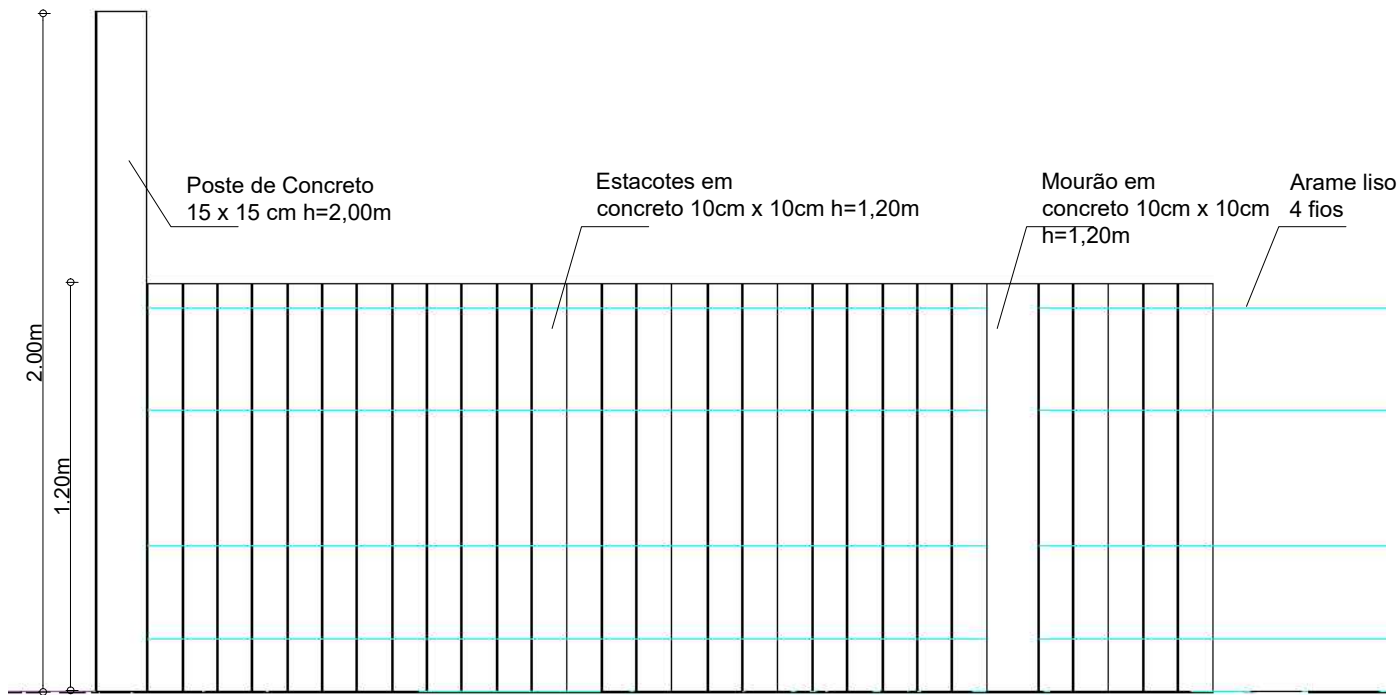
VISTA 1 - CERCA DE ESTACOTE ESC.: 1/25
