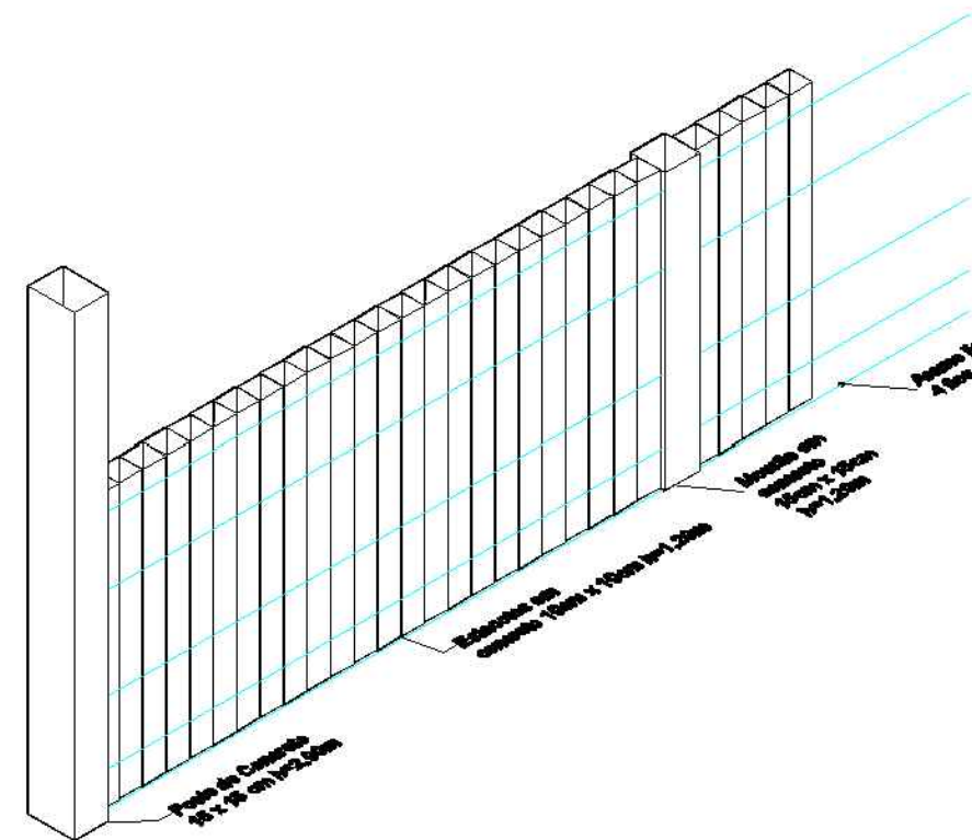
ISOMÉTRICA - CERCA DE ESTACOTE SEM ESCALA
