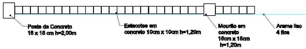
PLANTA - CERCA DE ESTACOTE ESC.: 1/25
