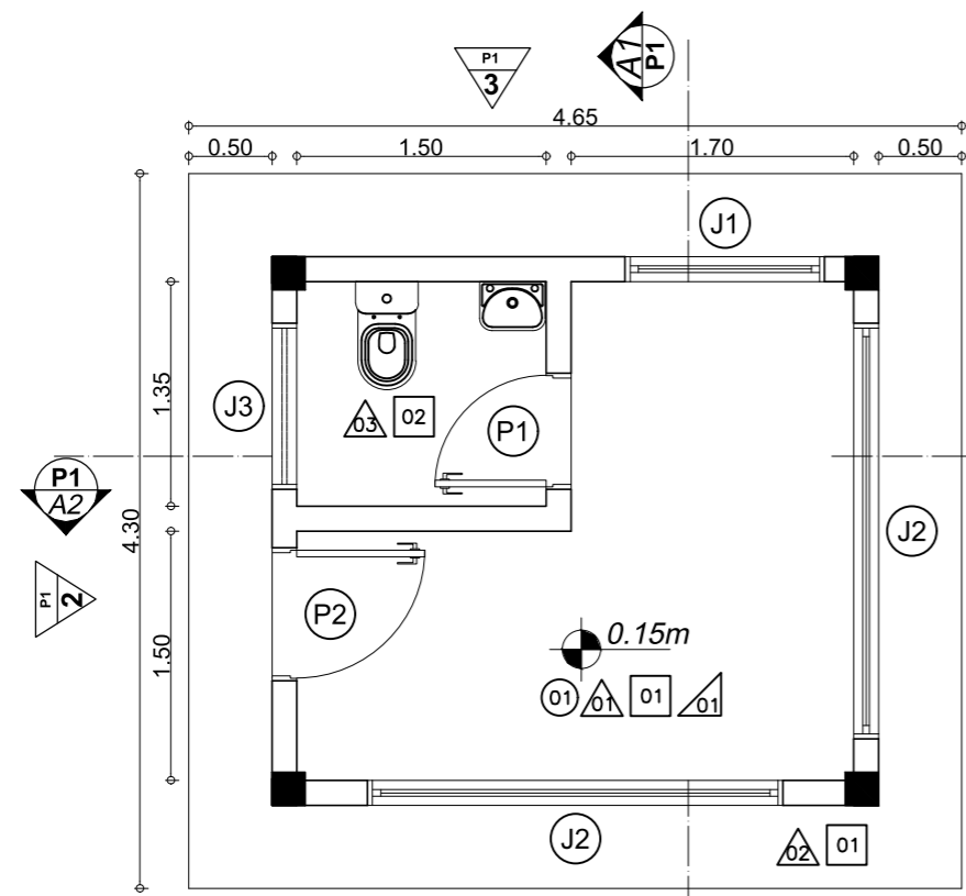
PLANTA BAIXA - GUARITA ESC.: 1/50
