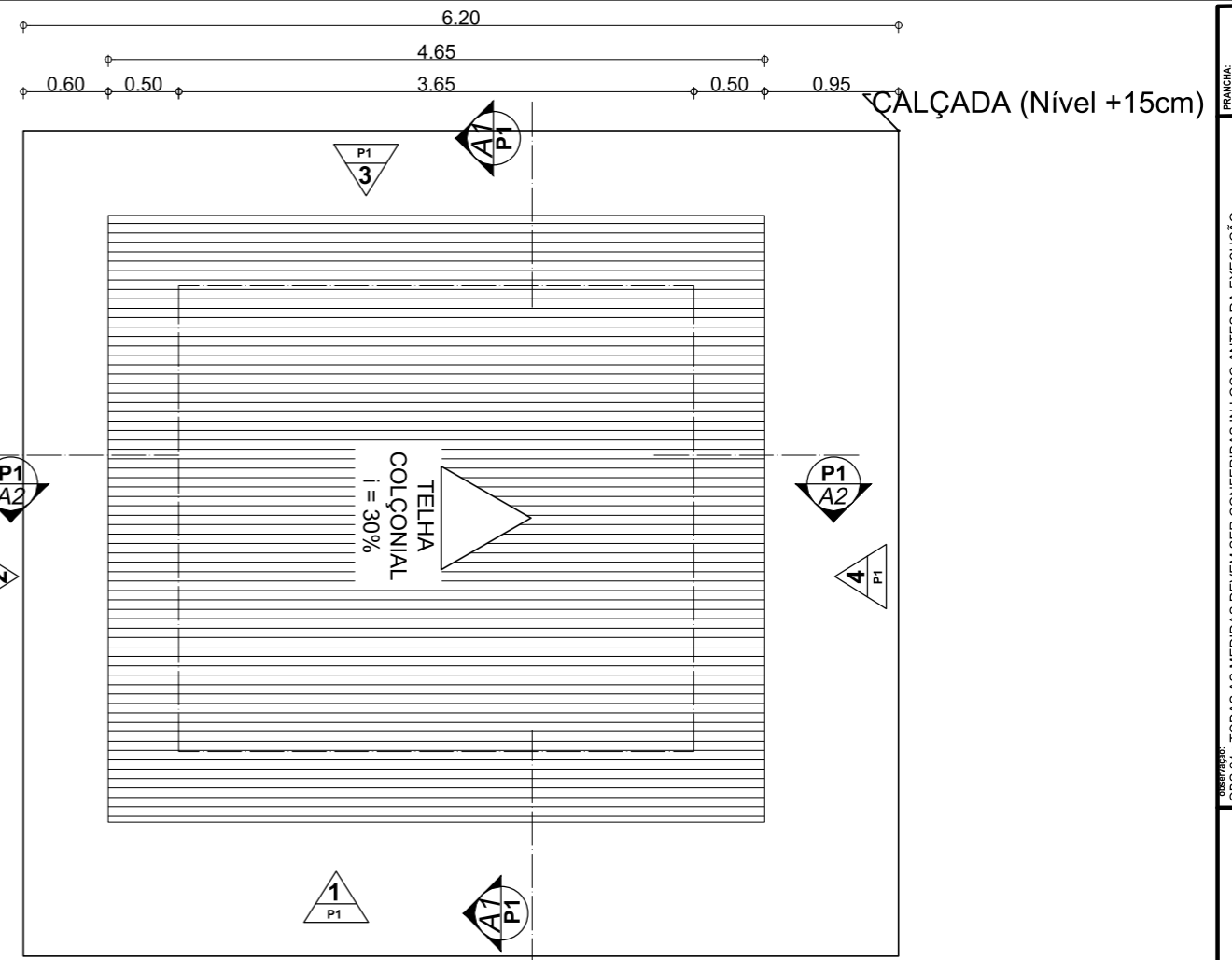
PLANTA DE COBERTA - GUARITA ESC.: 1/50
