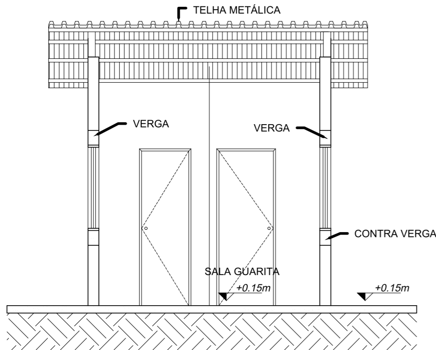
CORTE A1 ESC.: 1/50
