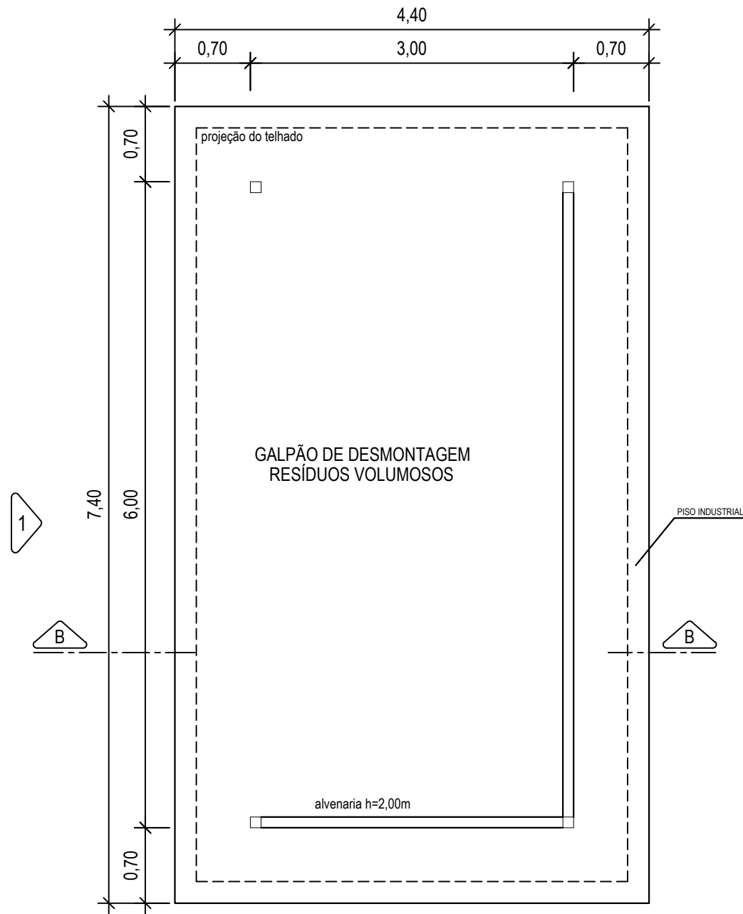
PLANTA BAIXA - GALPÃO DE DESMONTAGEM DE RESÍDUOS VOLUMOSOS ESC.: 1/50
