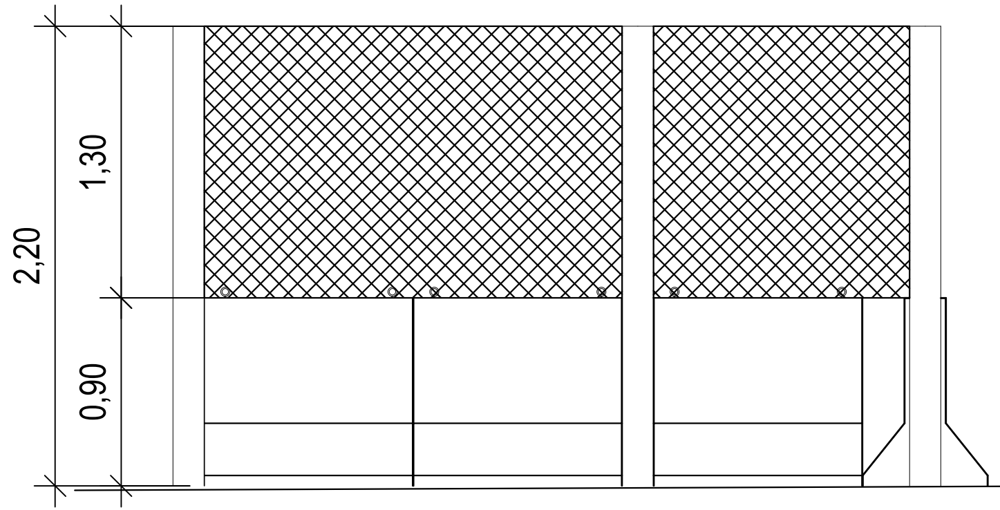
VISTA 2 ESC.: 1/25
