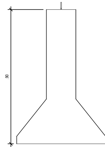
VISTA 2 ESC.: 1/75
