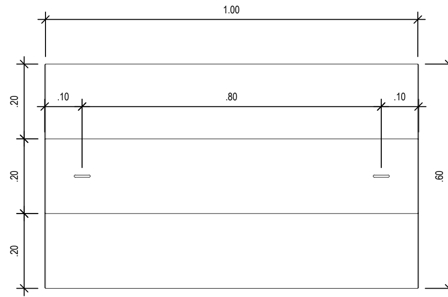
PLANTA BAIXA - BLOCO ESC.: 1/75
