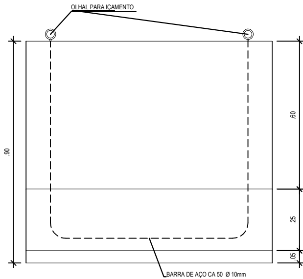
VISTA 1 ESC.: 1/75
