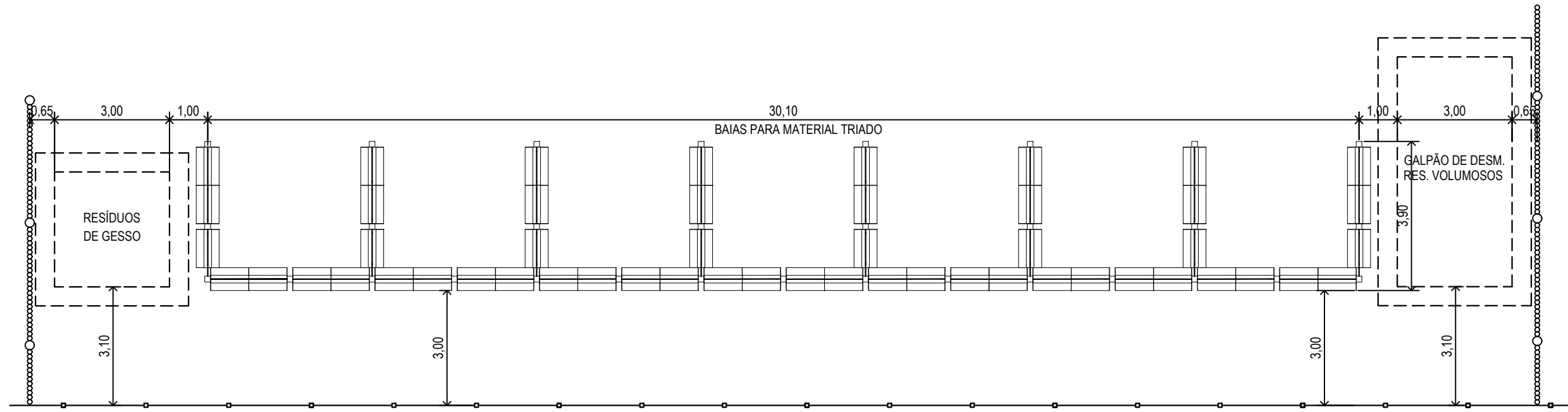
LOCAÇÃO DAS INSTALAÇÕES DA TRIAGEM ESC.: 1/125
