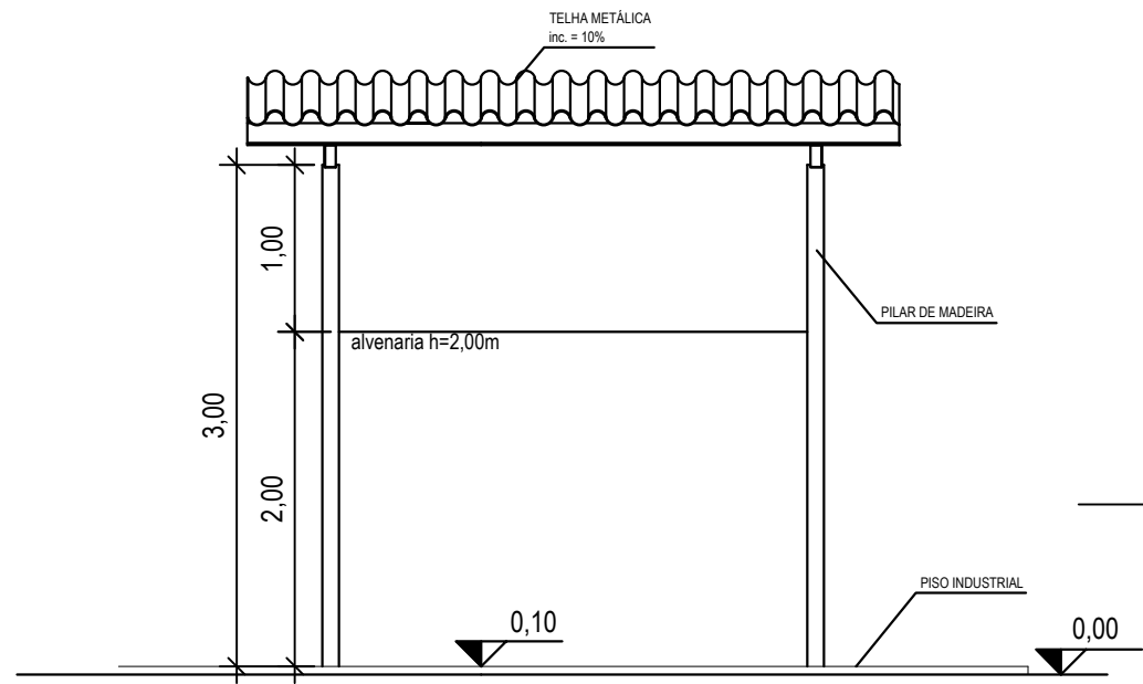
VISTA 2 - RESÍDUOS DE GESSO ESC.: 1/50
