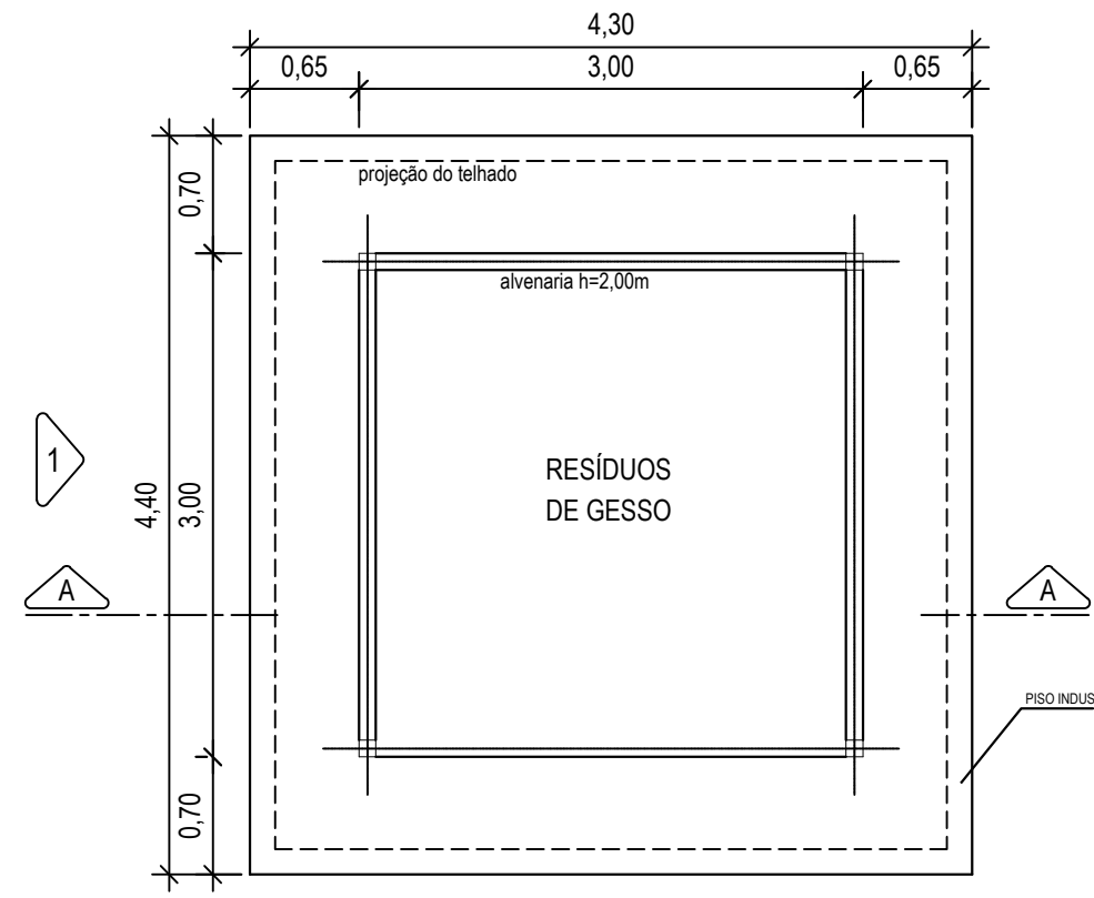
PLANTA BAIXA - RESÍDUOS DE GESSO ESC.: 1/50
