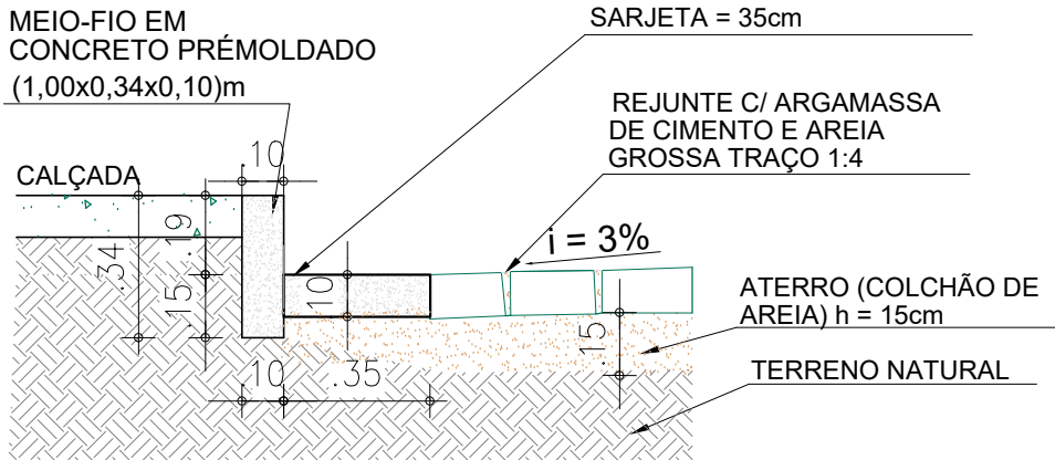
2 DETALHE SARJETA
