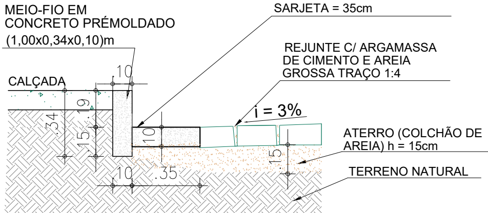
2 DETALHE SARJETA
